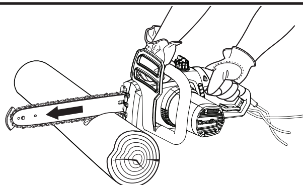
COUPE PAR LE DESSUS
