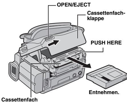
Cassettenfach
