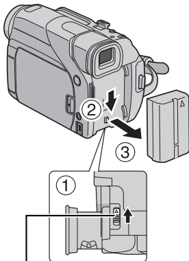
BATT.RELEASE
