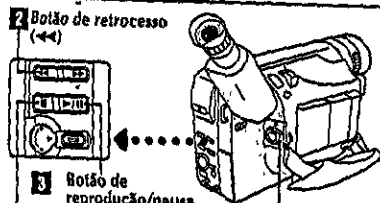
Botão de parar (■)
