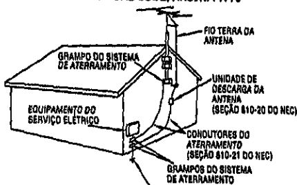
EXEMPLO DE ATERRAMENTO DE ANTENA, SEGUNDO O NATIONAL ELECTRICAL CODE, ANSI/NFPA 70
