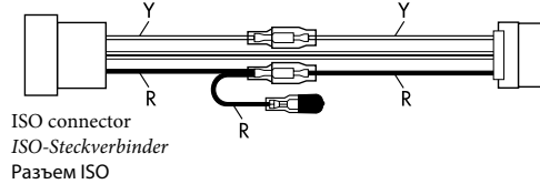
Original wiring / Original verdrahtung / Исходная схема соединений
