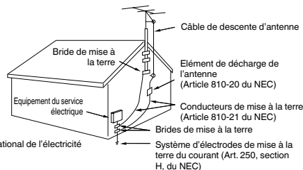
EXEMPLE DE LA MISE À LA TERRE DE L'ANTENNE SELON LES INSTRUCTIONS DU CODE DE L'ÉLECTRICITÉ
