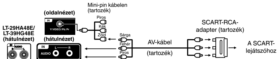
Csatlakozás SCART-lejátszóhoz
