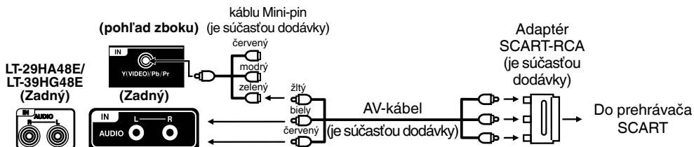
Prípojenie k prehrávaču SCART
