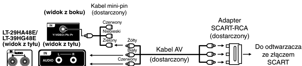
Podłączanie odtwarzacza ze złączem SCART
