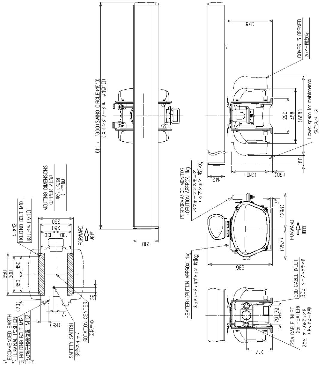
SCANNER UNIT OUTLINE DRAWING NOTE: Diameter of cable gland is not able to change. (注) ケーブルグランド径は変更できません。 SCNKE5302
