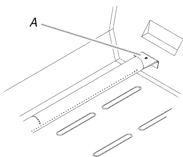
A. 2 tornillos
