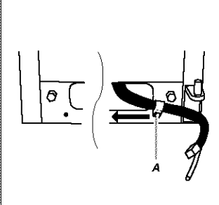
A. Abrazadera de la manguera
