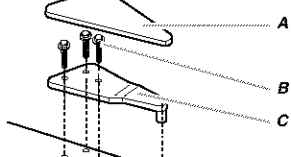
A. Tapa de la bisagra superior B. Tornillos de cabeza hexagonal para bisagra de 5/16" C. Bisagra superior
