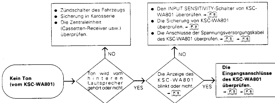
Tafel 1. Den Betrieb ohne Reproduktion von Ton überprüfen.
