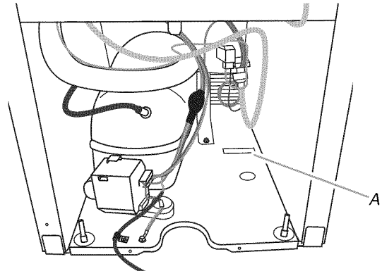
A. Ranura de la lengüeta de montaje
