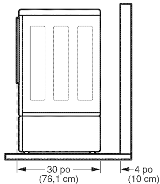
Dimensions requises pour installation avec piédestal
