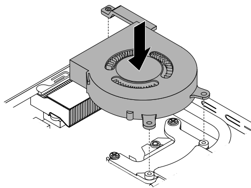
図 43. システム・ファンの取り付け (M700 および M900 の場合)
