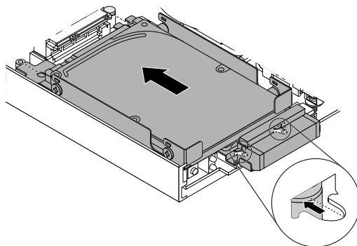
図 53. ストレージ・ドライブ・ブラケットの取り付け
