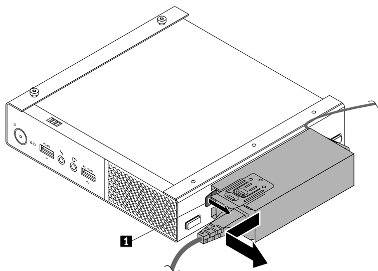
図 33. 電源アダプター・ブラケットの取り外し
