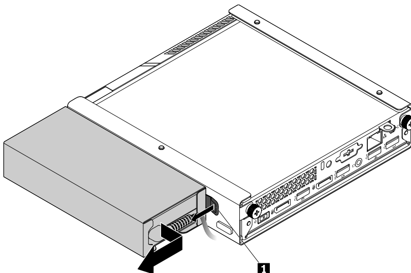
図 35. 電源アダプター・ブラケットの取り外し
