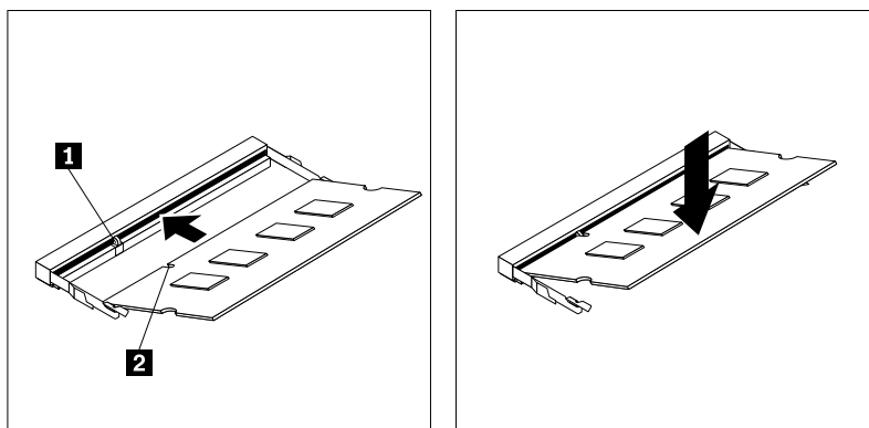
図 60. メモリー・モジュールの取り付け
