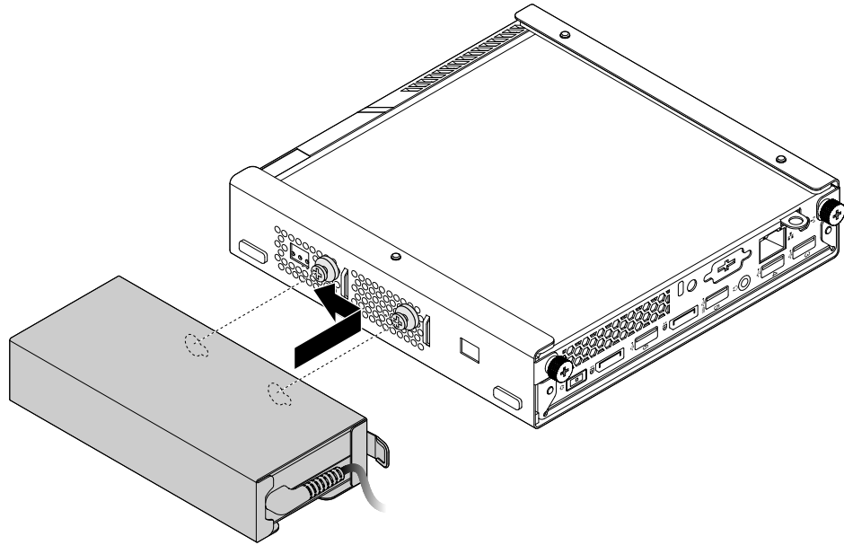
図 36. 電源アダプター・ブラケットの取り付け
