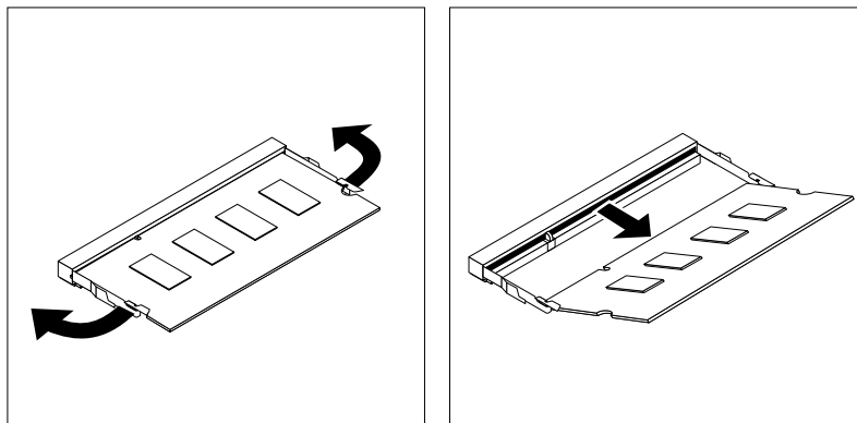
図 59. メモリー・モジュールを取り外す
