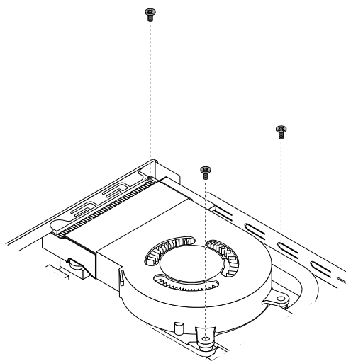
図 45. システム・ファンのねじの取り付け (M700 および M900 の場合)
