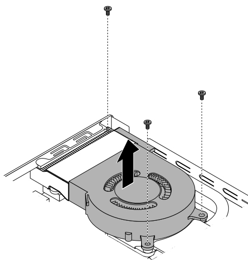
図 41. システム・ファンの取り外し (M700 および M900 の場合)
