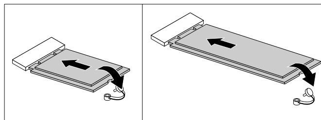
図 57. M.2 ストレージ・ドライブの取り付け
