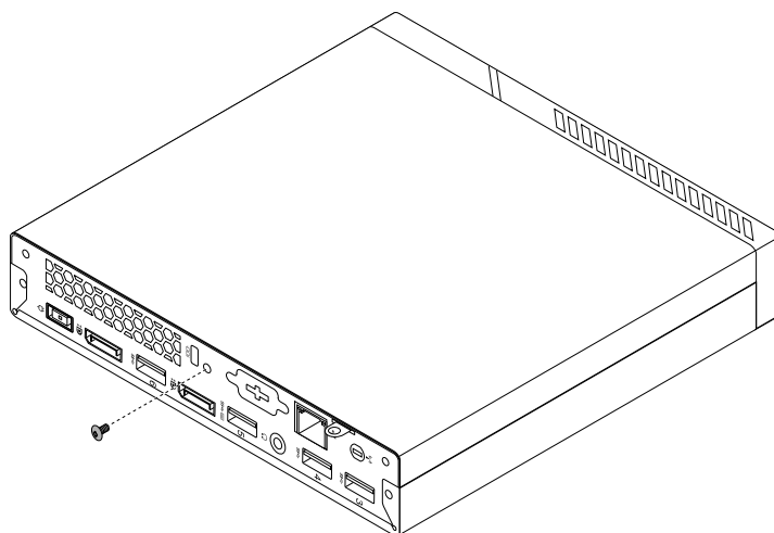
図 38. コンピューター・カバーのねじの取り外し
