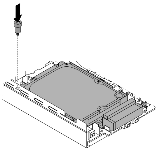
図 54. ストレージ・ドライブ・ブラケットのねじの取り付け
