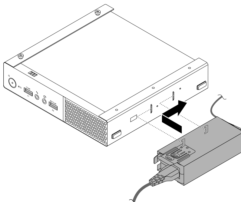
図 34. 電源アダプター・ブラケットの取り付け
