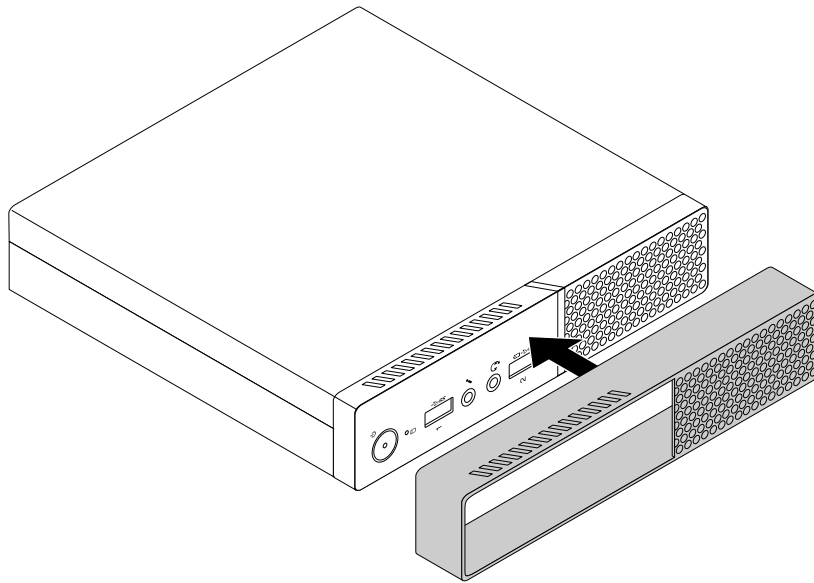
図 68. ダスト・シールドの取り付け
