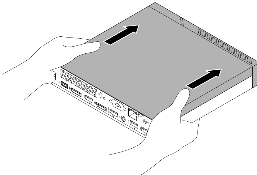
図 39. コンピューターのカバーの取り外し
