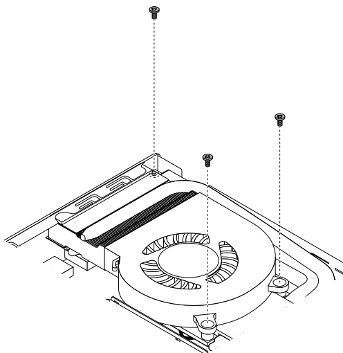
図 46. システム・ファンのねじの取り付け (M900x の場合)
