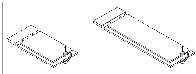
図 55. M.2 ストレージ・ドライブのねじの取り外し
