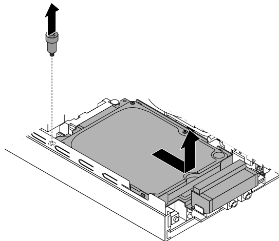
図 50. ストレージ・ドライブ・ブラケットの取り外し
