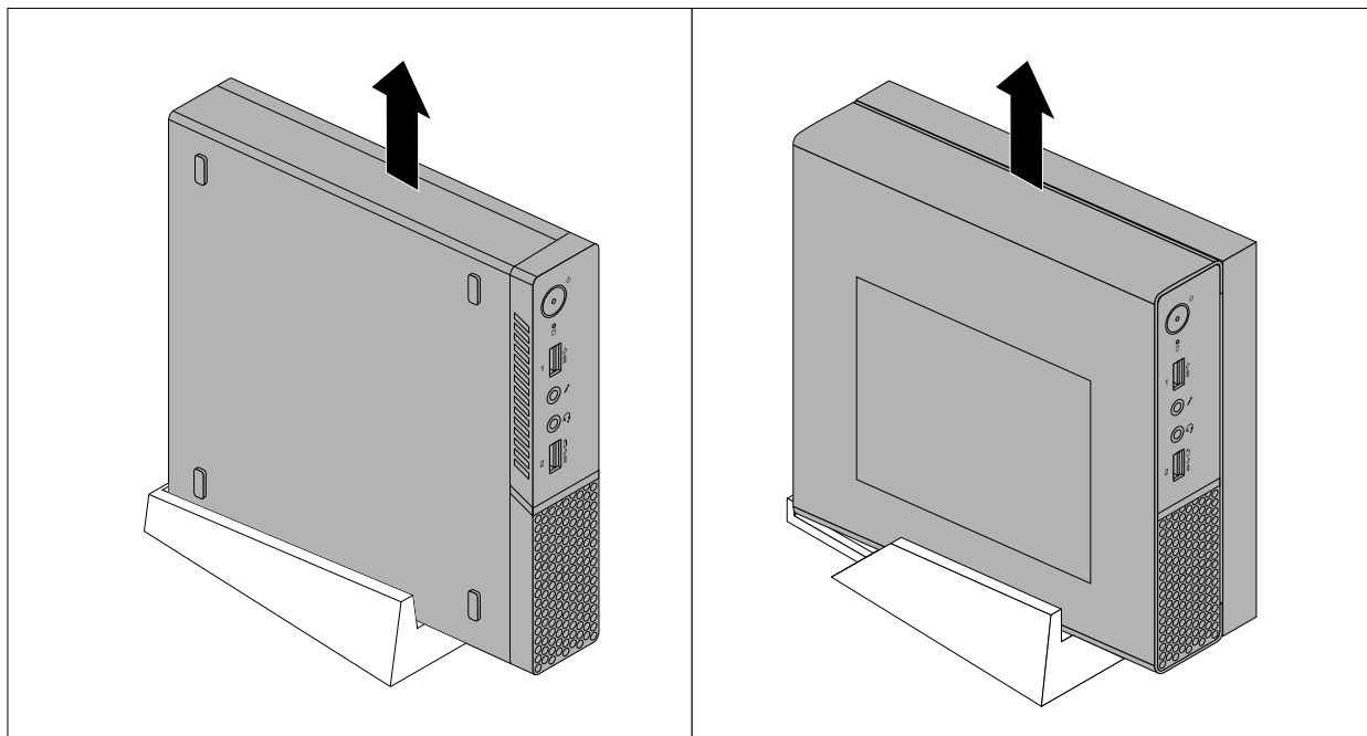
図 11. 縦置きスタンドからのコンピューターの取り外し
