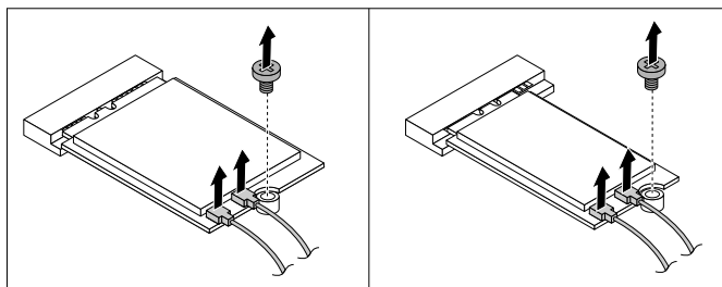
図 63. Wi-Fi カード・ケーブルの取り外し
