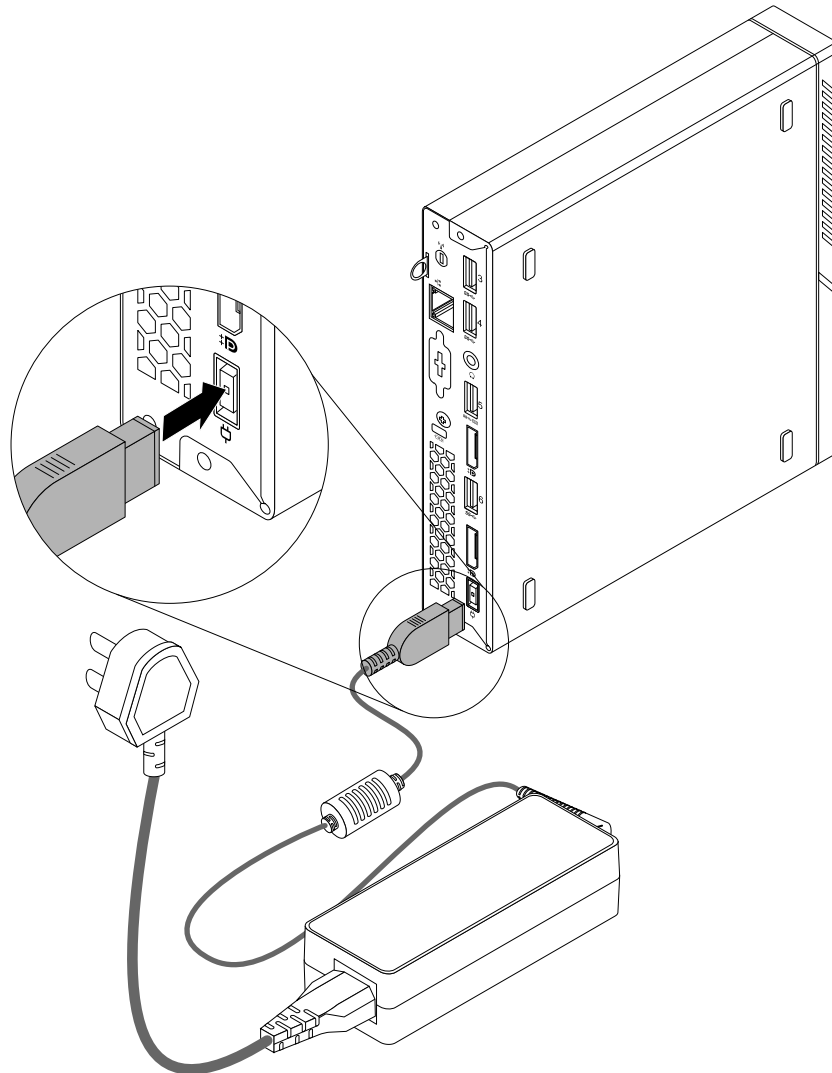
図 10. 電源アダプターの取り付け
