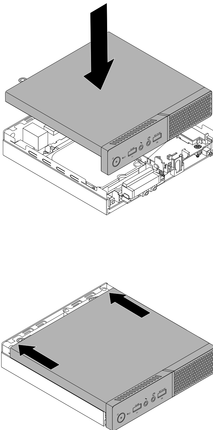
図 67. コンピューターのカバーの取り付け
