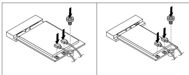
図 66. Wi-Fi アンテナ・ケーブルの接続
