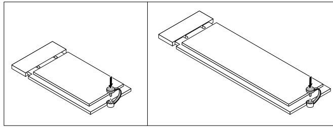
図 58. M.2 ストレージ・ドライブのねじの取り付け
