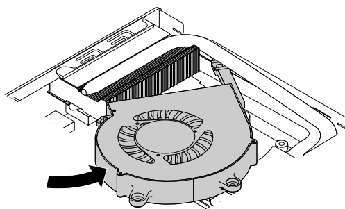
図 44. システム・ファンの取り付け (M900x の場合)
