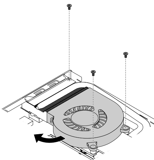
図 42. システム・ファンの取り外し (M900x の場合)
