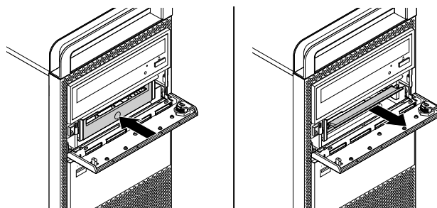
図 23. 3.5 型ストレージ・ドライブストレージ・ドライブ・ブラケットの取り外し
