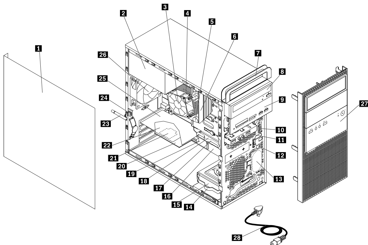
図3. コンピューターの構成部品
