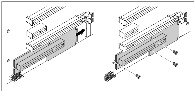
図 41. PCI アダプター・カードの取り付け
