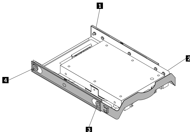
図 17. 2.5 型ストレージ・コンバーターの 3.5 型ストレージ・ドライブ・ブラケットへの取り付け
