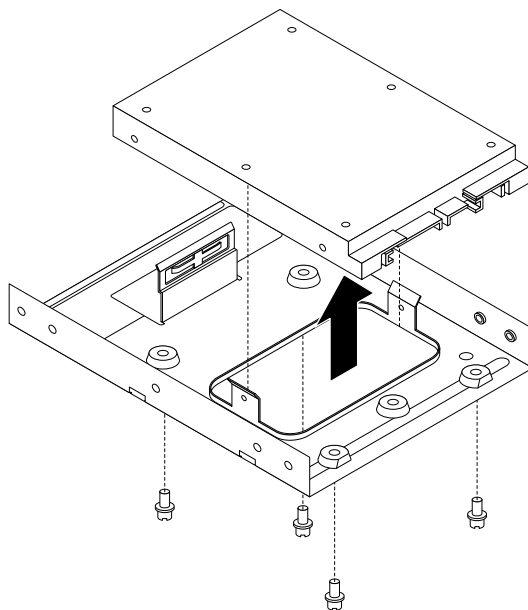
図 15. 2.5 型ストレージ・ドライブのストレージ・コンバーターからの取り外し
