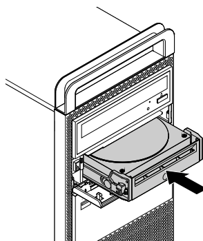
図26. フロントアクセス・ストレージの筐体への 3.5 型ストレージ・ドライブ・ブラケットの取り付け
