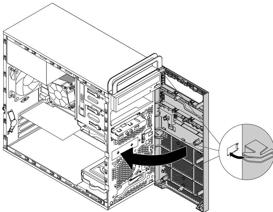
図 12. 前面ベゼルの取り付け
