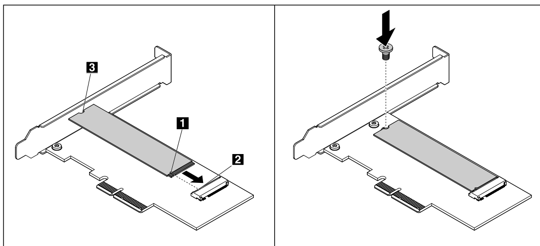
図 29. M.2 ソリッド・ステート・ドライブの取り付け
