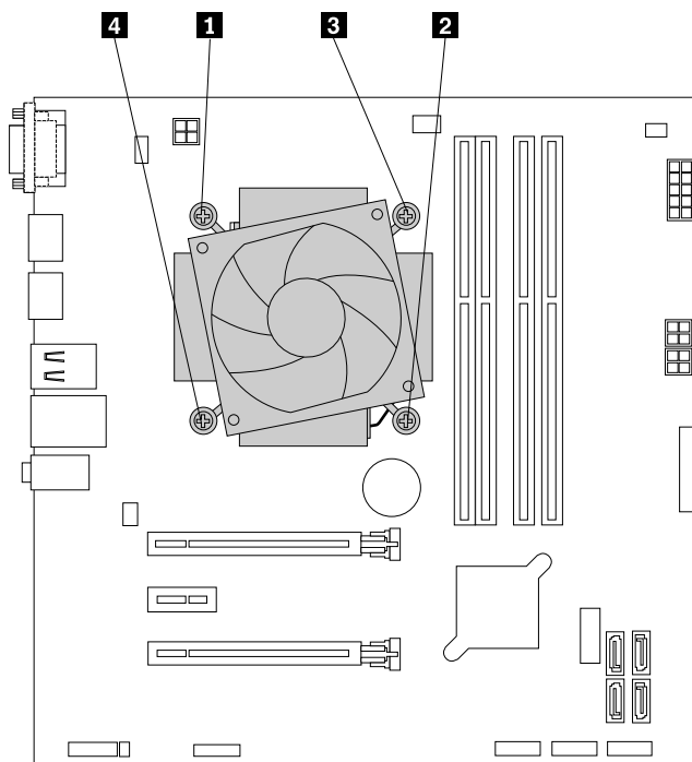
図34. ヒートシンクとファン・アセンブリーの取り外し
