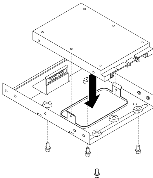
図 16. 2.5 型ストレージ・ドライブのストレージ・コンバーターへの取り付け
