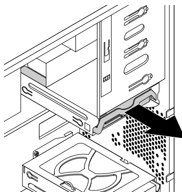
図 14. 3.5 型ストレージ・ドライブストレージ・ドライブ・ブラケットの取り外し
