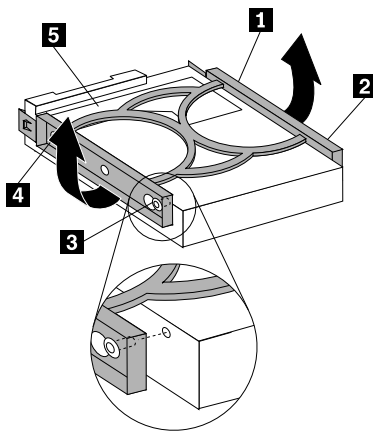
図 20. 3.5 型ストレージ・ドライブのブラケットへの取り付け
