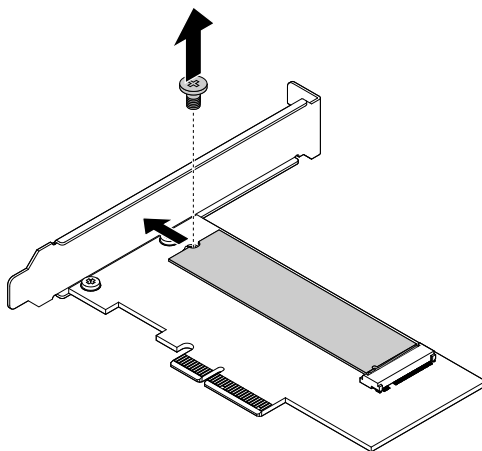
図 28. M.2 ソリッド・ステート・ドライブの取り外し
