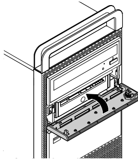
図 27. 3.5 型ストレージ・ドライブ・ブラケットの固定
