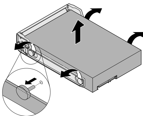
図 24. ブラケットからの 3.5 型ストレージ・ドライブの取り外し
