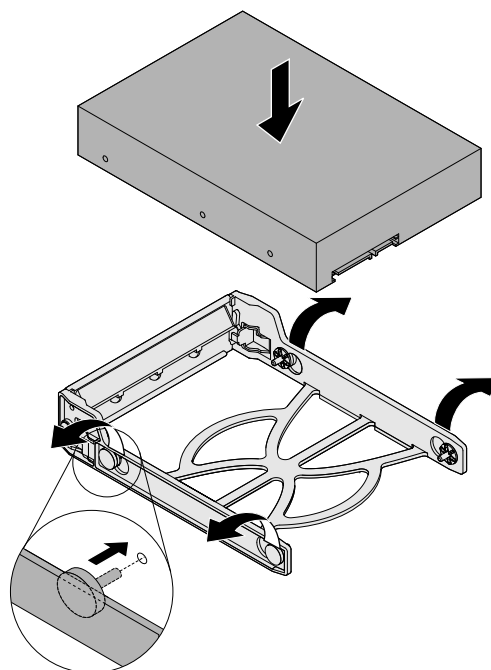
図25. 3.5 型ストレージ・ドライブのブラケットへの取り付け
