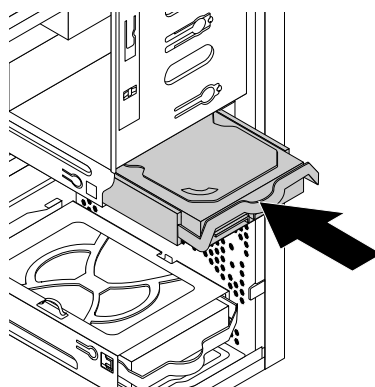
図 18. 3.5 型ストレージ・ドライブ・ベイの取り付け
