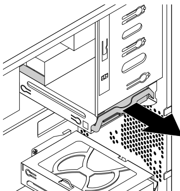
図 19. 3.5 型ストレージ・ドライブストレージ・ドライブ・ブラケットの取り外し
