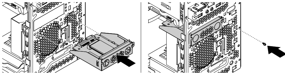
图 65. 将转换装置连同 mSATA 固态硬盘一并装入机箱
