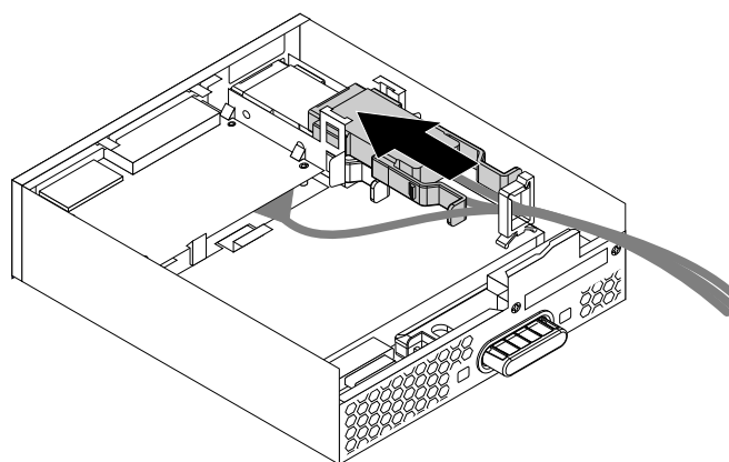
图 39. 将 eSATA 接口或 IEEE 1394 接口装入 Flex 模块
