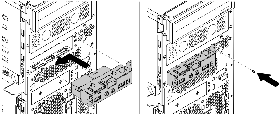
图 52. 安装正面音频和 USB 组合件
