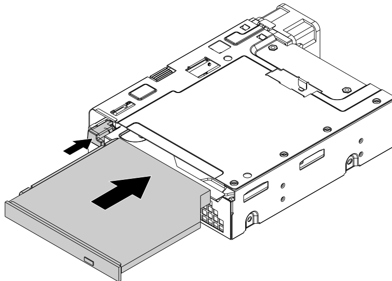
图 44. 将薄型光盘驱动器装入 5.25 英寸保持架组合件
