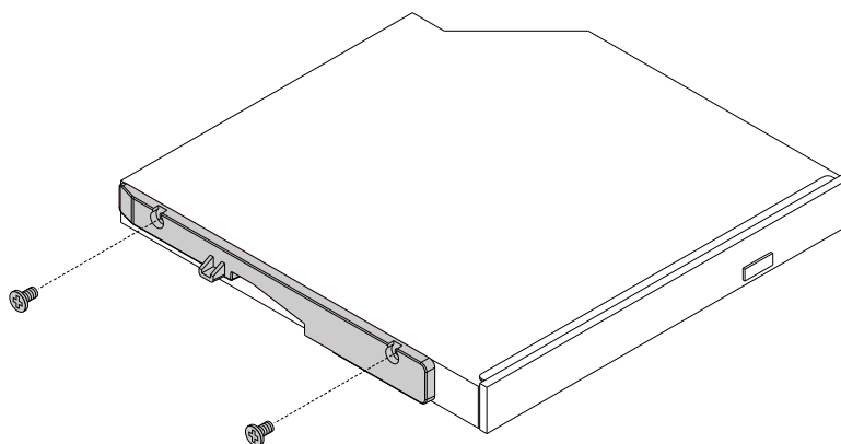
图 42. 卸下薄型光盘驱动器固定器
