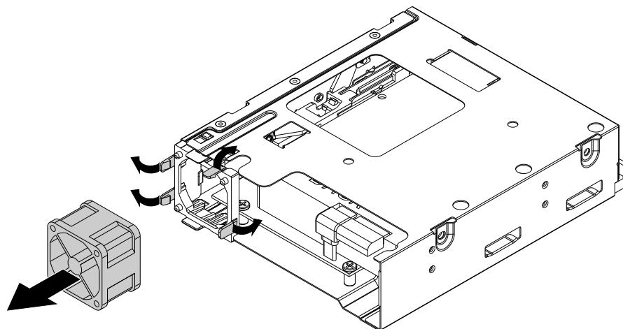
图 47. 从 5.25 英寸保持架组合件上卸下风扇
