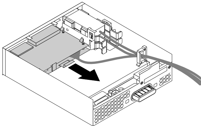
图 32. 卸下 Flex 模块中的读卡器
