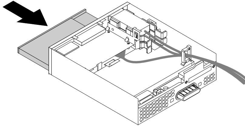
图 29. 将薄型光盘驱动器装入 Flex 模块
