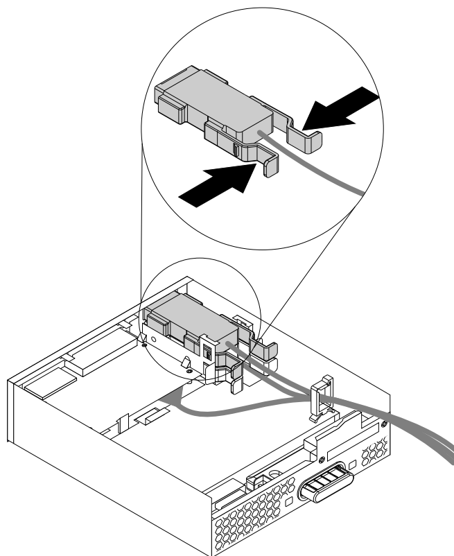
图 38. 卸下 Flex 模块中的 eSATA 接口或 IEEE 1394 接口
