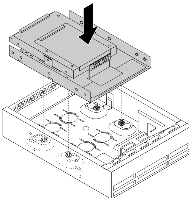
图 80. 安装固态驱动器和转换装置
