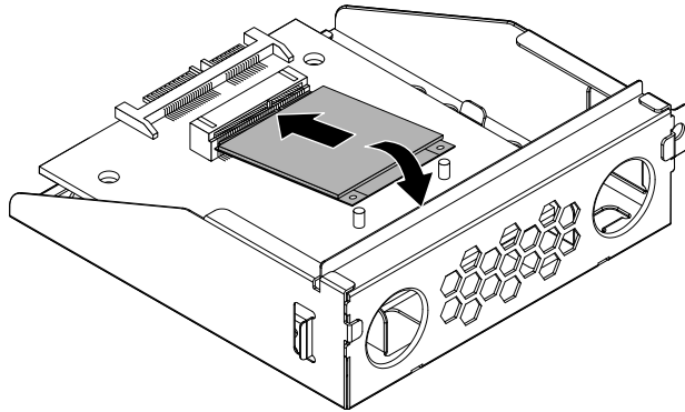
图 69. 将 mSATA 固态硬盘装入转换装置中
