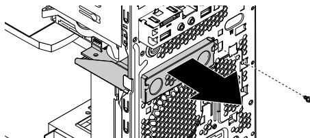
图 66. 将转换装置连同所安装的 mSATA 固态硬盘一并卸下
