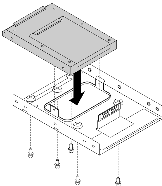
图 79. 将固态驱动器装入转换装置中
