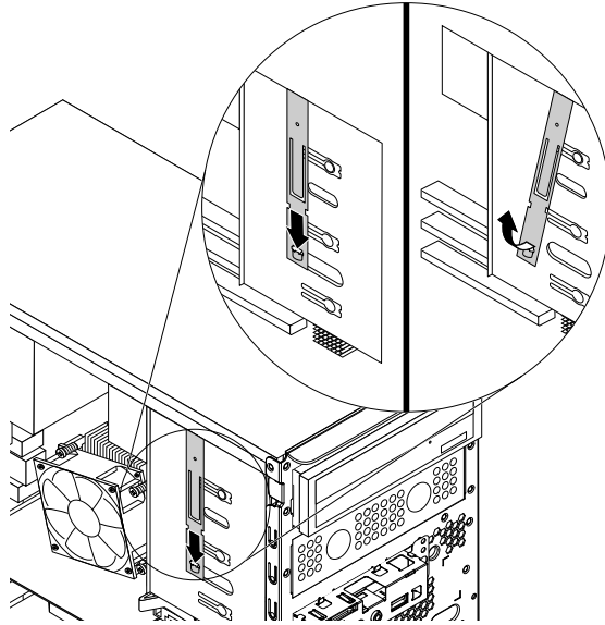
图 19. 从计算机上卸下光盘驱动器固定器
