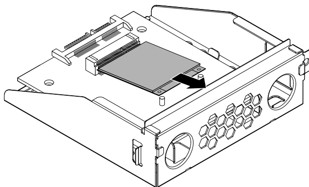
图 68. 从转换装置上卸下 mSATA 固态硬盘
