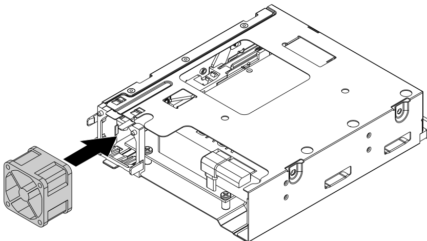
图 48. 将风扇装入保持架组合件
