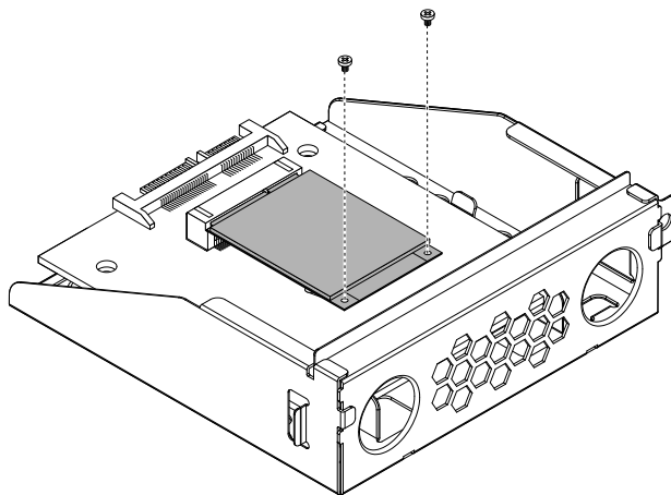
图 67. 卸下固定 mSATA 固态硬盘的螺钉
