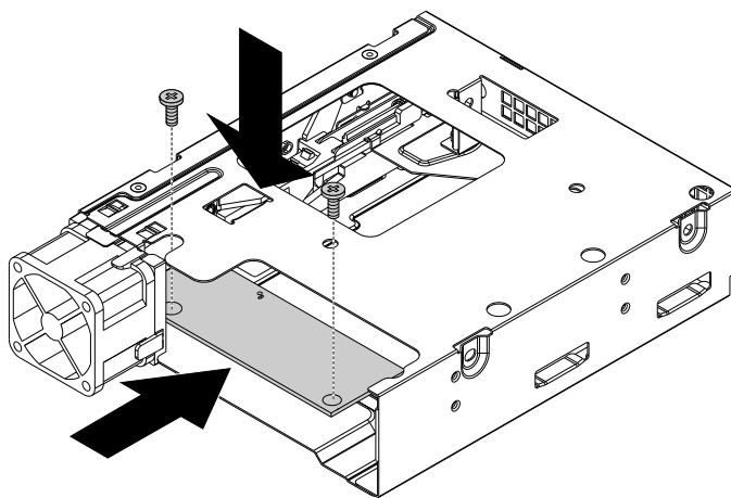
图 50. 安装薄型光盘驱动器转换板
