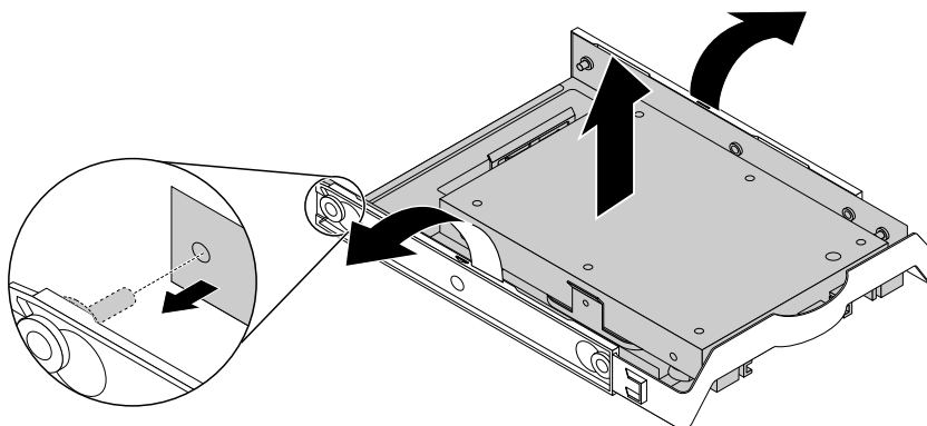
图 59. 从 3.5 英寸硬盘驱动器支架上卸下转换装置
