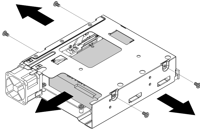
图 45. 从 5.25 英寸保持架组合件上卸下硬盘驱动器
