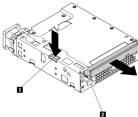
图 41. 卸下 5.25 英寸保持架组合件中的薄型光盘驱动器
