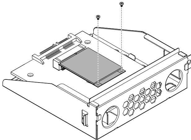
图 70. 安装螺钉以固定 mSATA 固态硬盘
