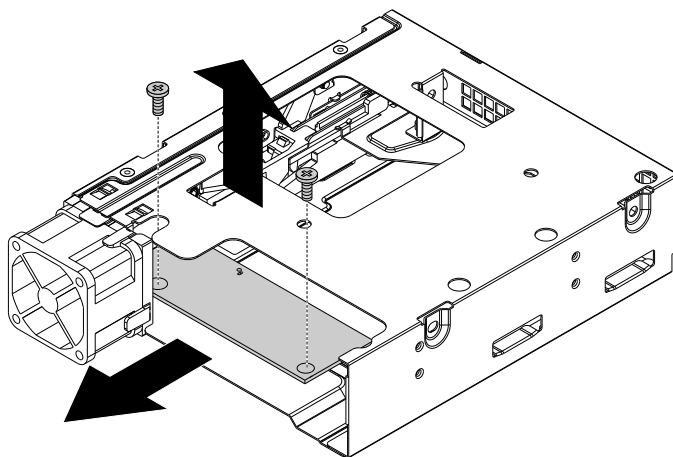
图 49. 卸下薄型光盘驱动器转换板
