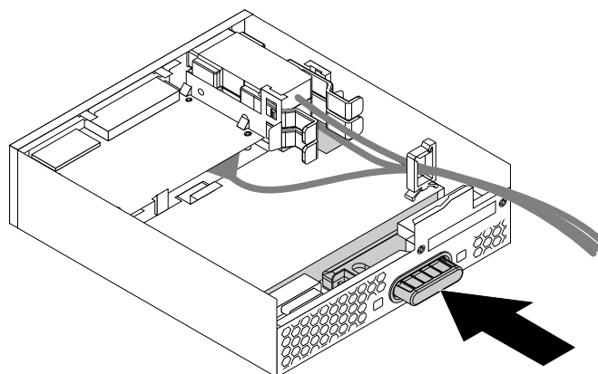
图 26. 从 Flex 模块上卸下薄型光盘驱动器
