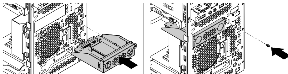
图 71. 安装 mSATA 固态硬盘
