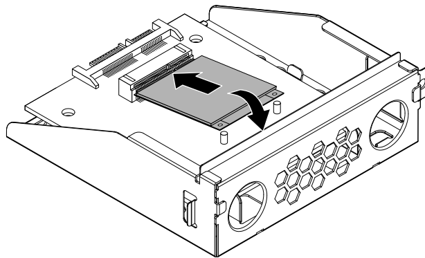
图 63. 将 mSATA 固态硬盘装入转换装置中
