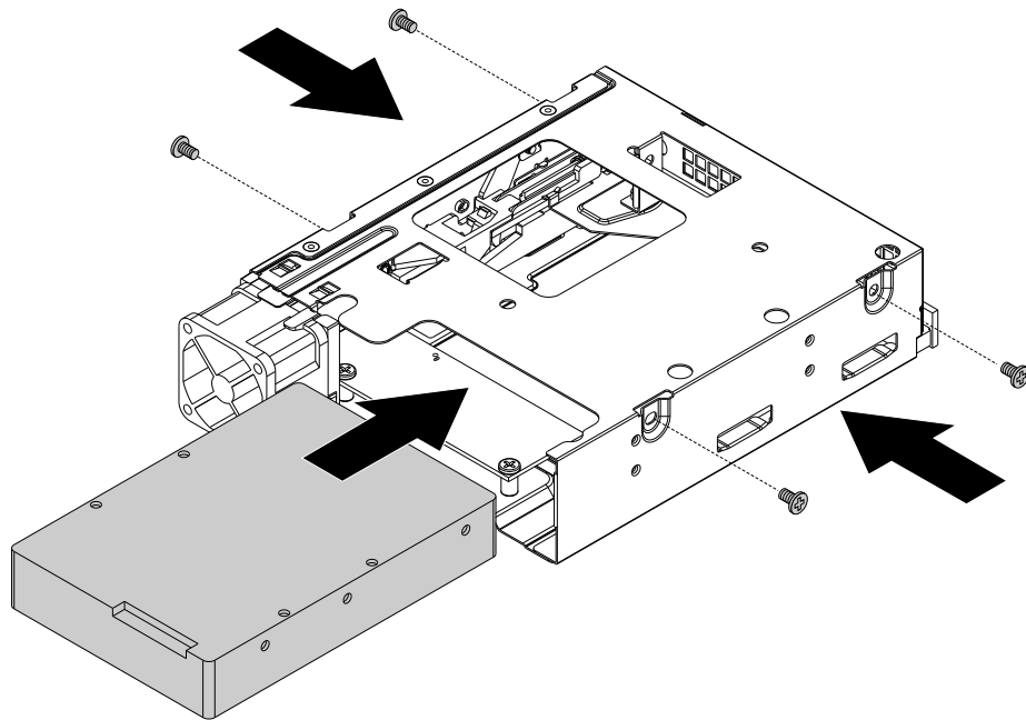
图 46. 将硬盘驱动器装入 5.25 英寸保持架组合件
