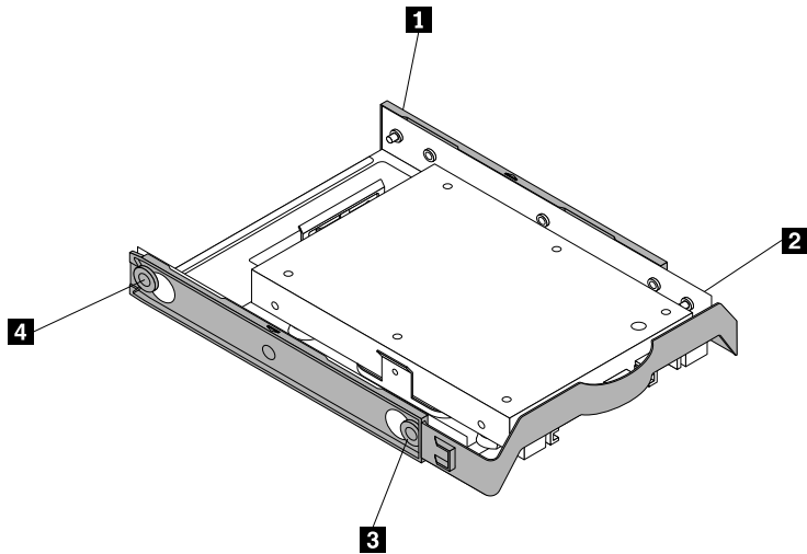
图 58. 将转换装置连同固态驱动器一并装入硬盘驱动器支架
