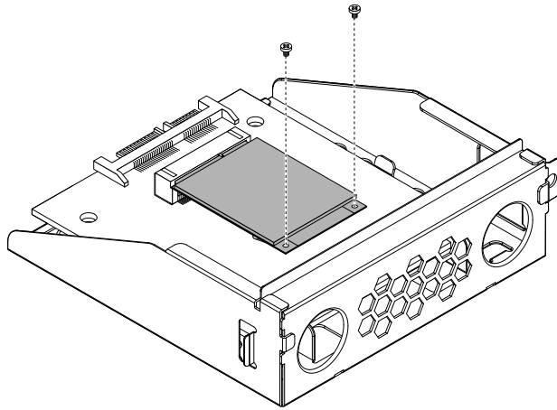
图 64. 安装螺钉以固定 mSATA 固态硬盘
