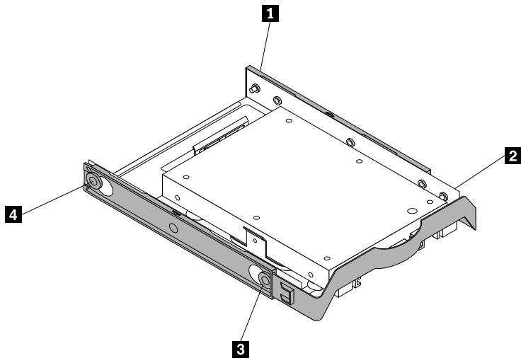
图 62. 将转换装置连同新的固态驱动器一并装入硬盘驱动器支架
