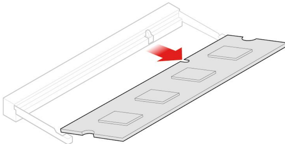
图 87. 卸下内存条
