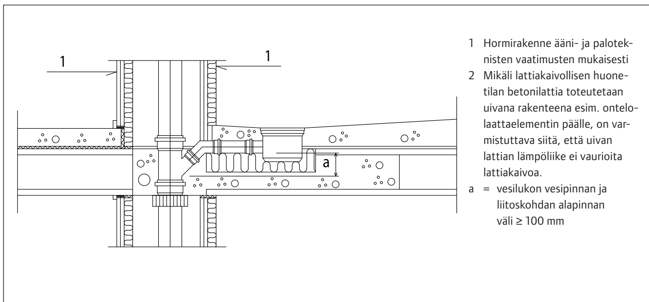
Kuva 82. Lattiakaivon kytkentäviemäriin liittäminen 45°-haarayhteellä pystykokojaviemäriin.
