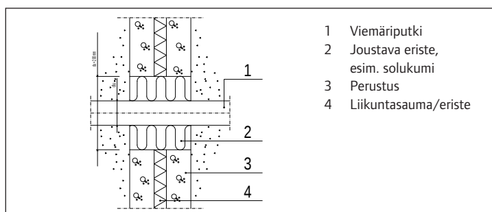
Kuva 47. Maahan asennetun viemäriputken läpivienti liikuntasäumallisen rakenteen läpi, palo-osastoimaton rakenne.
