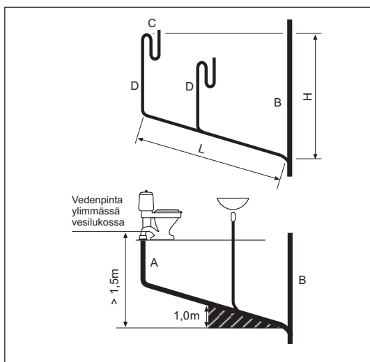
Kuva 38. Tuulettamattoman kokoojaviemärin mitoitus.
