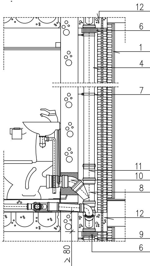
Kuva 7. Esimerkki levyrakenteisesta seinärakenteesta eristämättömän Uponor-kiinteistöviemärin yhteydessä äänitasovaatimuksella 33 dB(A). EI 30.
