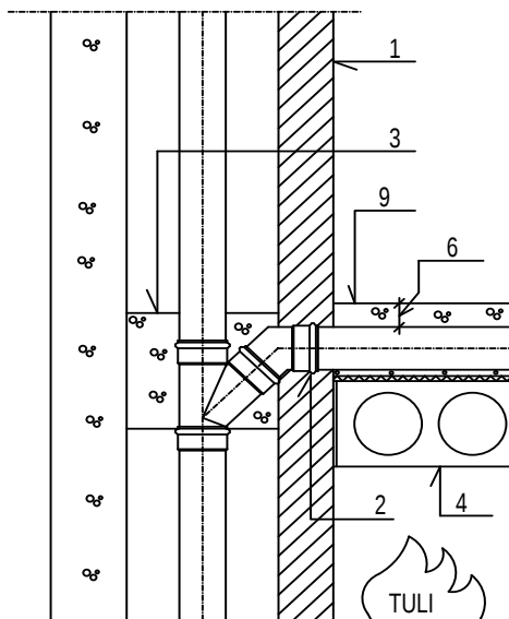
A. Uponor-kiinteistöviemärin palo-osastointi pystykokoojaviemärin suojarakenteella, vaakaviemäri betonivalussa.
