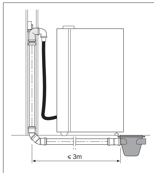
Kuva 83. Pesukoneen liittäminen viemäriverkostoon viemärintikulmalla ja kulmaliittimellä.
