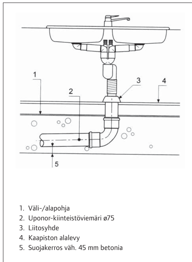
Kuva 81. Astianpesualtaan liittäminen viemäriin liitosyhteen avulla.
