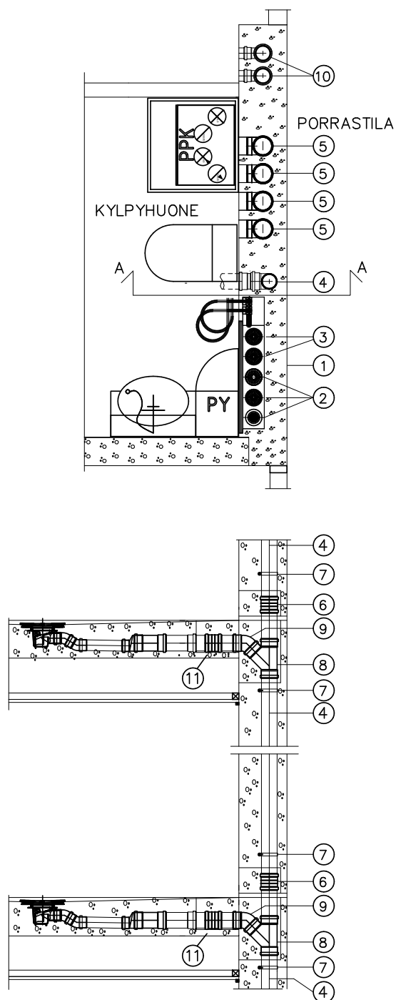
LEIKKAUS A - A
