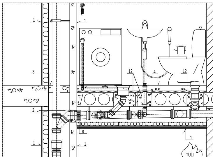
J. Uponor-kiinteistöviemärin palo-osastointi pystykokoojaviemärin suojarakenteella ja suojarakenteen lävistävällä vaakaviemärissä olevalla palomansetilla. Vaakaviemärit välipohjan alapuolella.
