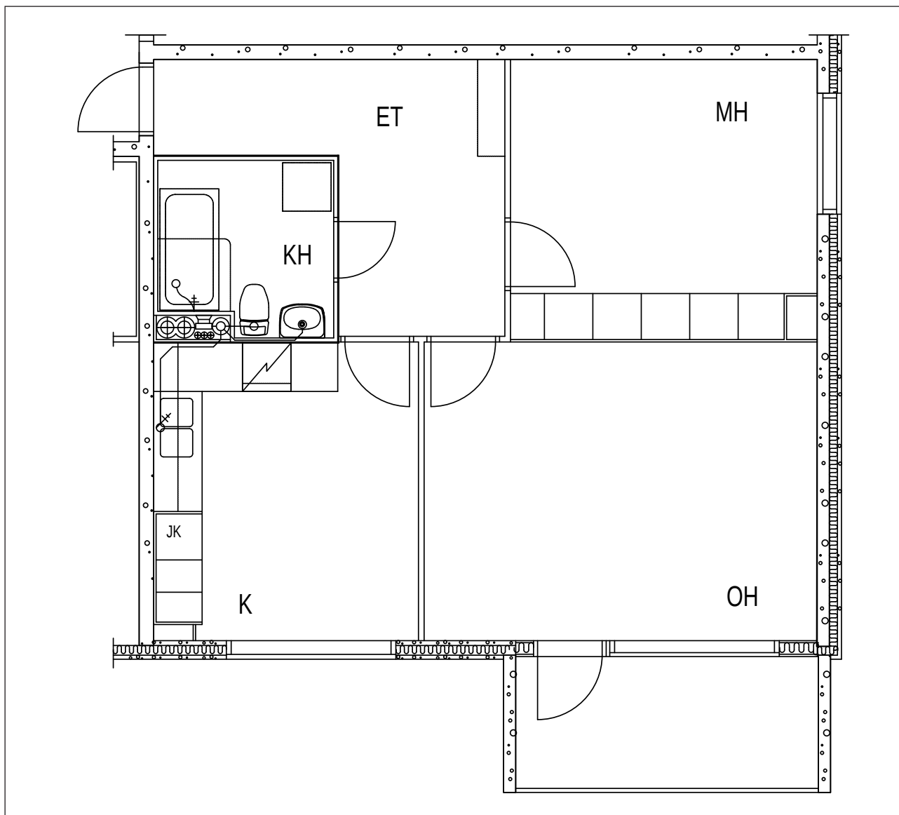
Kuva 49. 1970-luvulla rakennetun asuin-kerrostalohuoneiston jätevesiviemäriverkoston nykytilanne ennen perusparannustoimenpiteitä. Kylpyhuoneessa viemärikaivona on käytetty seinäkaivoa.
