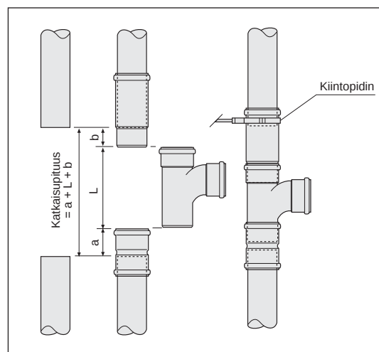
Kuva 64. Haaroitus haarayhteen, kaksoismuhvin ja liitos-/paisuntayhteen avulla.
