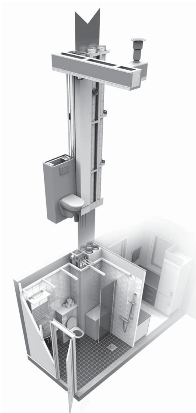
Kuva 57. B5-vaakaviemäri- ja B2-seinä-WC-elementit osana elementtiryhmittä.
