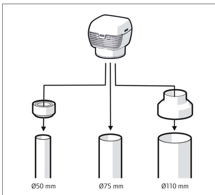
Kuva 112. Alipaineventtiilin asennus Uponor-kiinteistöviemäriputkeen.
