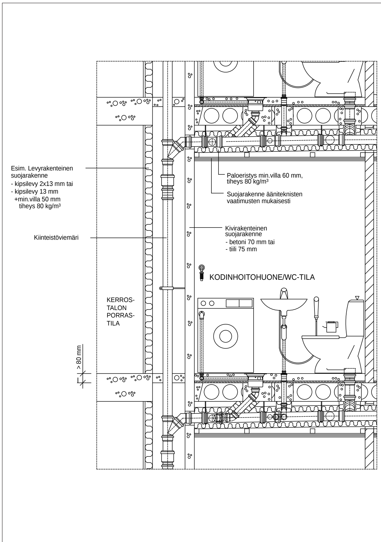
Kuva 30. Uponor-pystykokooviemärin palo-osastointi pystyviemärin suojarakenteella ja vaakaviemärin paloeristyksellä.
