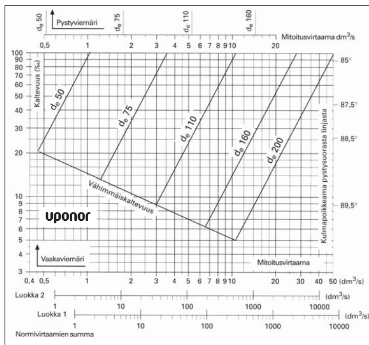
Kuva 39. Uponor-kokoojaviemäriin mitoitusdiagrammi.
