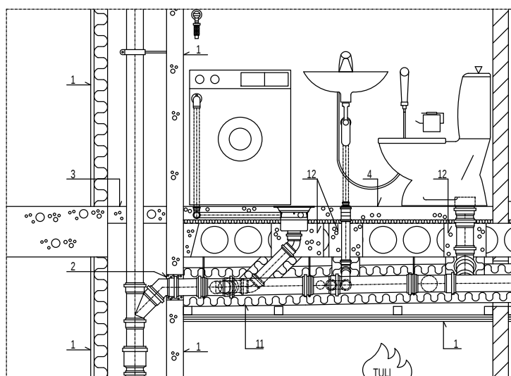
K. Uponor-kiinteistöviemärin palo-osastointi pystykokoojaviemärin suojarakenteella ja suojarakenteen lävistävän vaakaviemärin paloeristämisellä. Vaakaviemärit välipohjan alapuolella.
