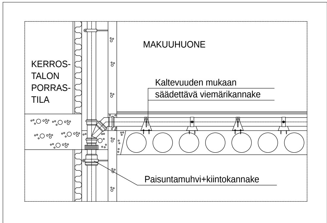
Kuva 74. Vaakaviemärin kannakointi ns. asennuslattiassa.
