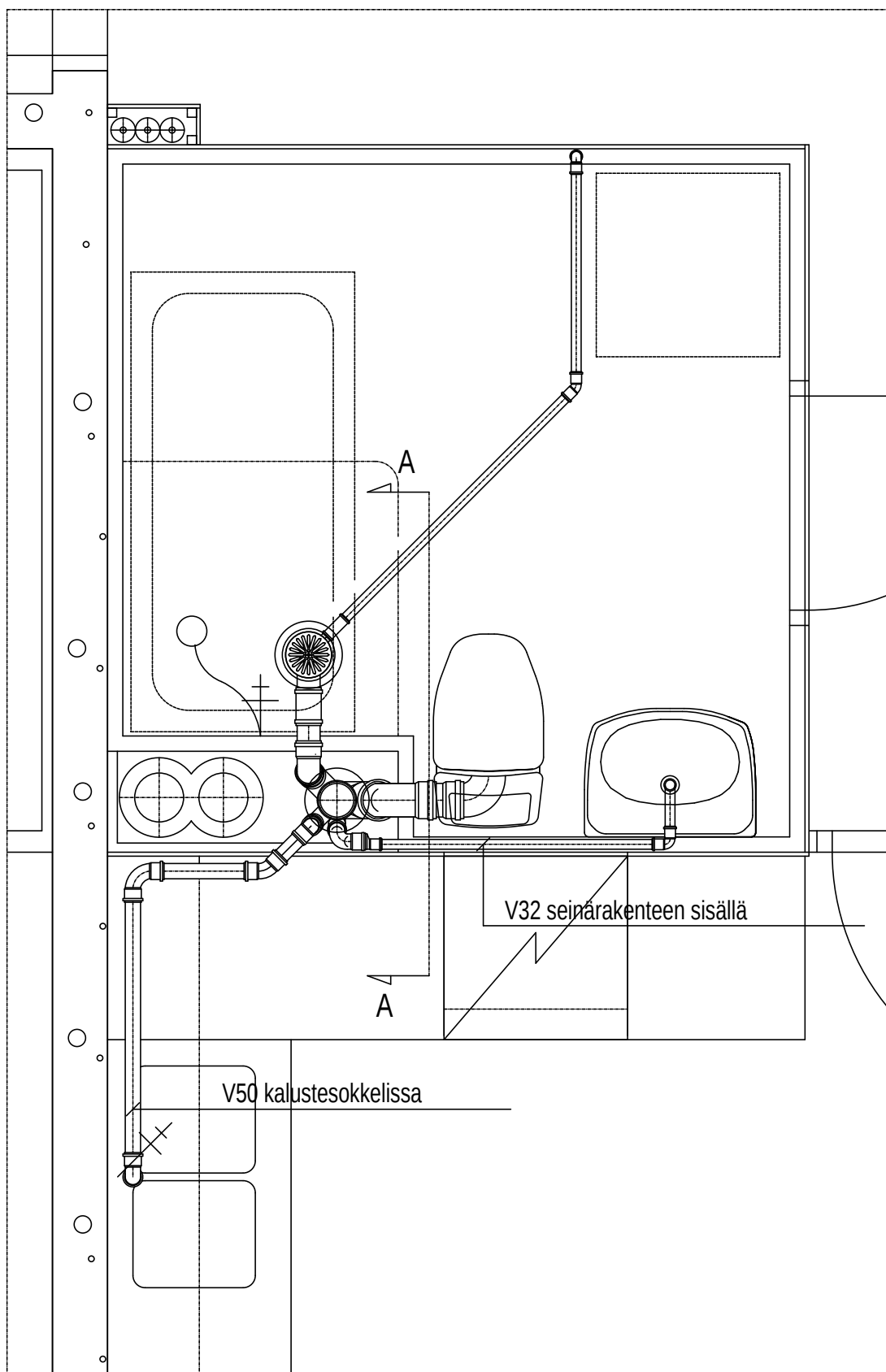
Kuva 61. 1970-luvulla rakennettu asuinkerrostalohuoneisto on perusparannettu Uponor-kiinteistöviemäreillä. Hormitila on rakennettu ääniteknisenä suojauksena tämän käsikirjan ohjeita noudattaen. Viemärin pohjakulmana on käytetty Uponor-pohjakulmaa.
