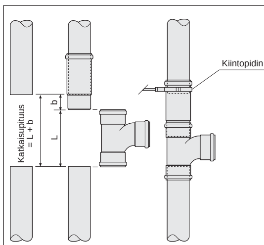
Kuva 63. Haaroitus muhvihaaran ja liitos-/paisuntayhteen avulla.
