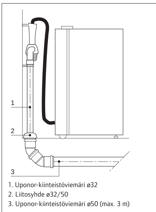
Kuva 84. Pesukoneen liittäminen viemäriverkostoon vesilukollisella pesukonesuppilolla.
