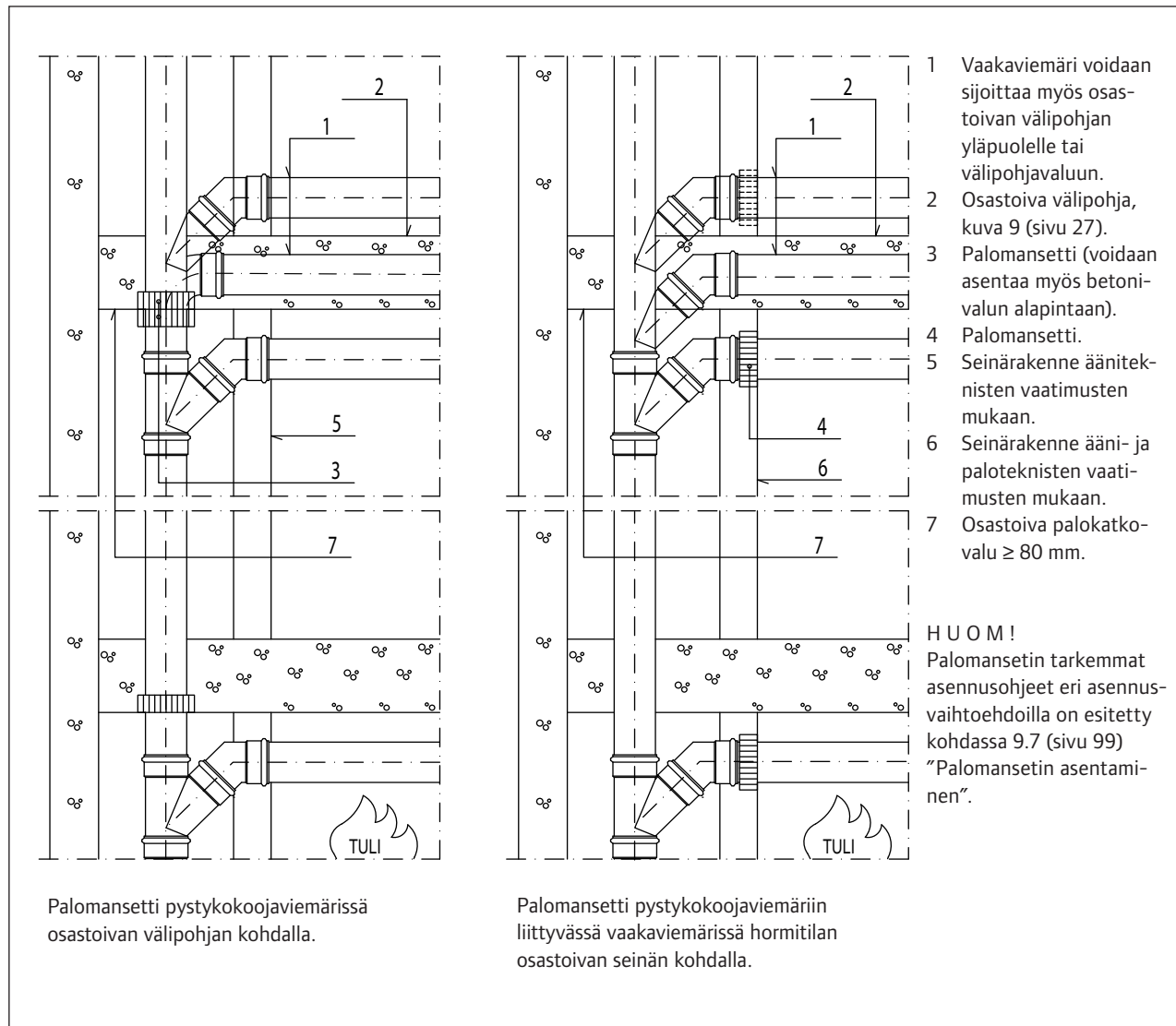
Kuva 27. Palomansetin sijoitusperiaate Uponor-kiinteistöviemärien yhteydessä.
