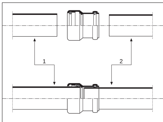
Kuva 65. Valurauta- ja Uponor-kiinteistöviemärien liittäminen jatkoyhteellä, jossa on kumitiiviste molemmille putkille (koot 75/70 ja 110/100 putkille).
