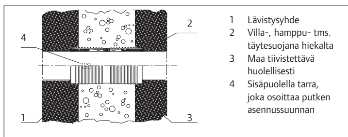
Kuva 48. Maahan asennetun viemäriputken läpivienti lävistysyhteellä, osastoimaton rakenne.
