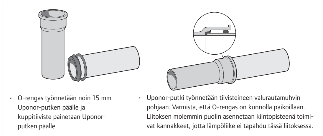
Kuva 66. Uponor-putken liittäminen valurautaviemäriin muhviin O-renkaan ja kuppitiivisteiden avulla.
