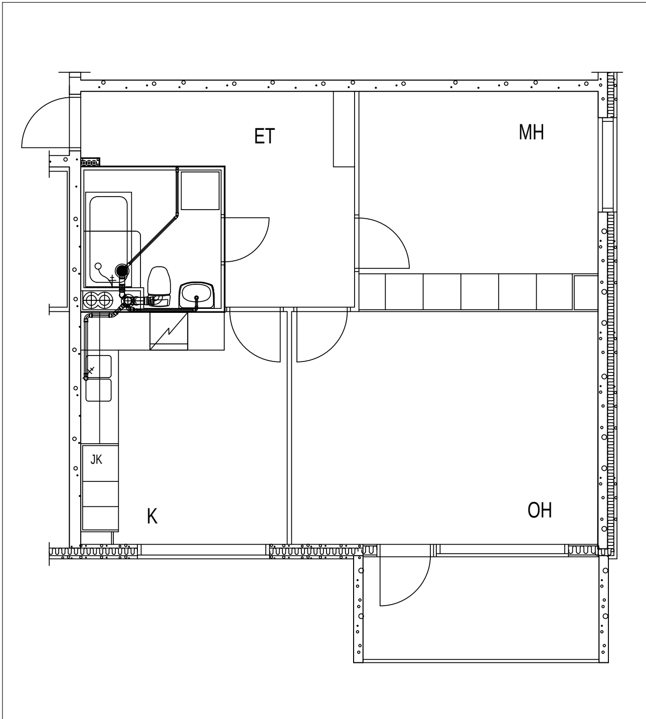
Kuva 60. 1970-luvulla rakennetun asuin-kerrostalo-ohuoneiston viemäriverkosto on perusparannettu Uponor-kiinteistöviemäreillä. Kylpyhuoneen seinäkaivo on korvattu lattiakaivolla.
