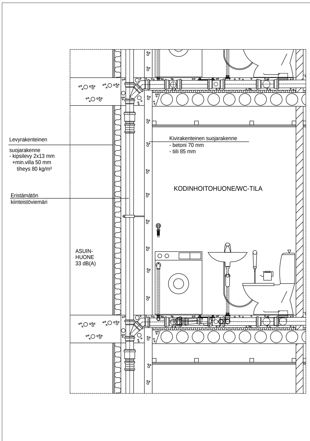
Kuva 2. Eristämättömän Uponor-kiinteistöviemärin äänitekniset suojarakenteet, äänitasovaatimus 33 dB(A).
