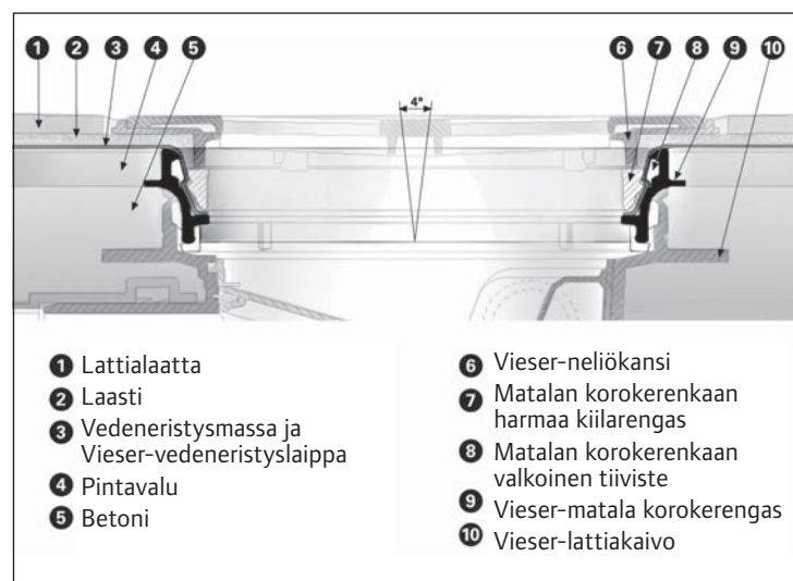
Kuva 98. Matalan korokerengaan asentaminen Vieser-lattiakaivoon.
