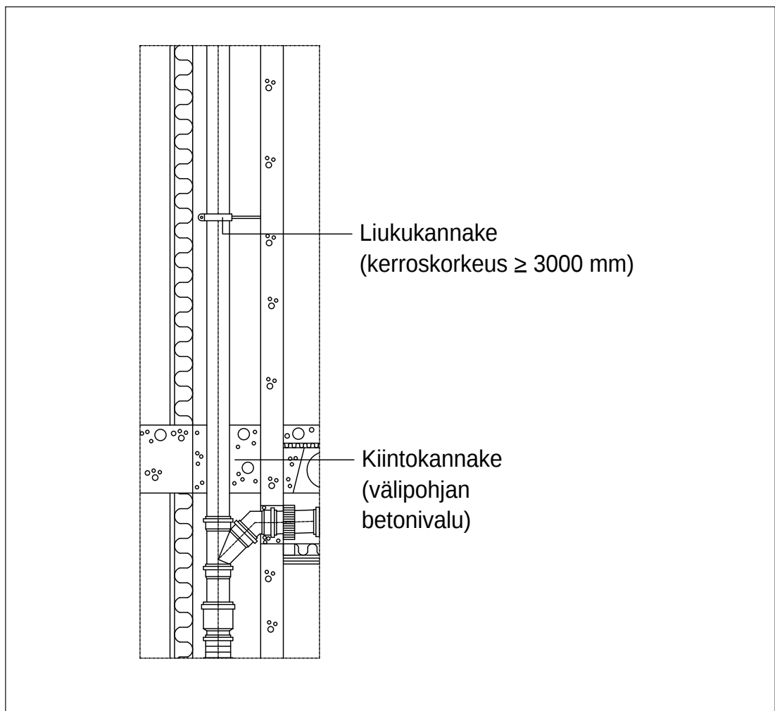
Kuva 75. Esimerkki pystyviemärin kannakoinnista.
