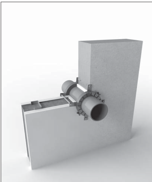
Kuva 106. Palomansetti rakenteen pintaan asennettuna. Kiinnitys palonkestävin ankkurein tai kevytseinässä läpikulutus.
