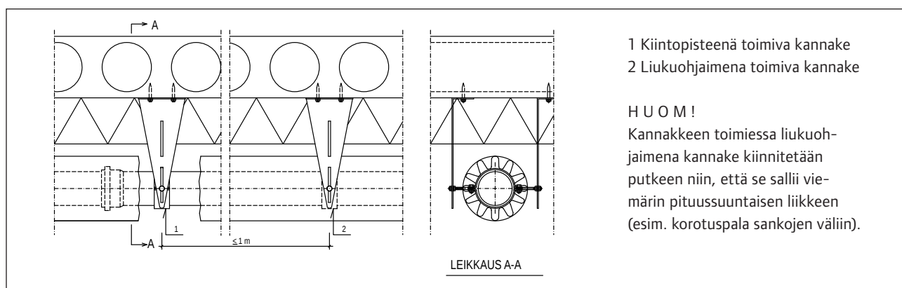
Kuva 72. Esimerkki vaakaviemärin kiintopisteestä.
