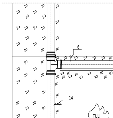
I. Uponor-kiinteistöviemärin palo-osastointi pystykokoojaviemärin ollessa betonisessa ELPO-elementissä. Vaakaviemäri betonisessa välipohjaelementissä.
