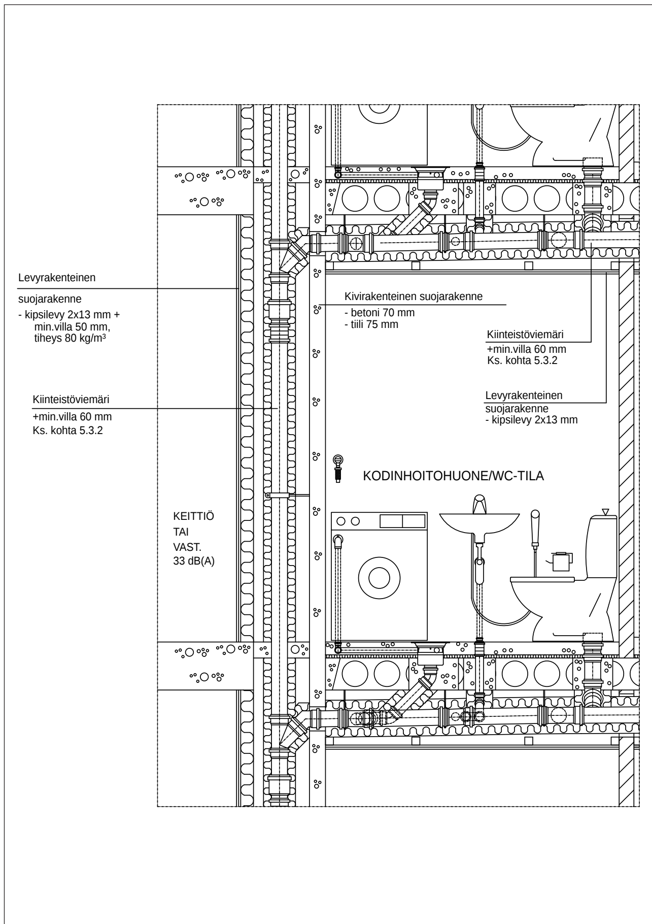
Kuva 4. Eristetyn Uponor-kiinteistöviemärin äänitekniset suojarakenteet, äänitasovaatimus 28 dB(A).
