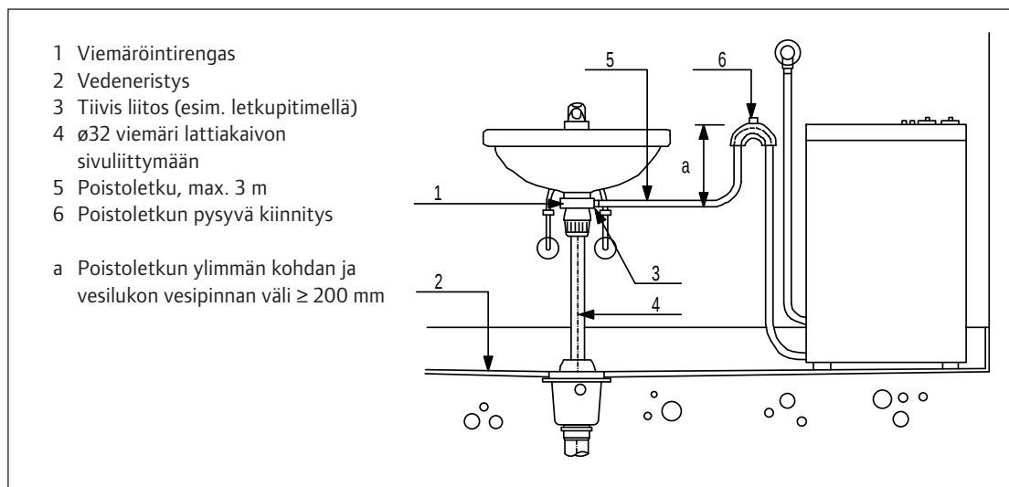
Kuva 91. Pesukoneen liittäminen viemäriverkostoon pesualtaan vesilukon yhteyteen asennetulla viemärintirengasella.
