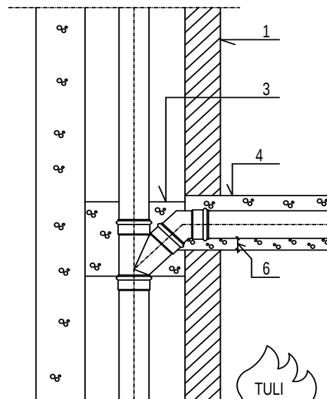
B. Uponor-kiinteistöviemärin palo-osastointi pystykokoojaviemärin suojarakenteella, vaakaviemäri betonirakenteisen välipohjan sisällä.
