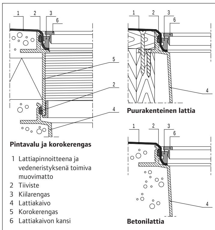
Kuva 99. Lattiakaivon ja vesieristyksen liittäminen.
