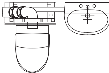
Kuva 55. seinä-WC-elementti V50 pesuallaskytkenällä.
