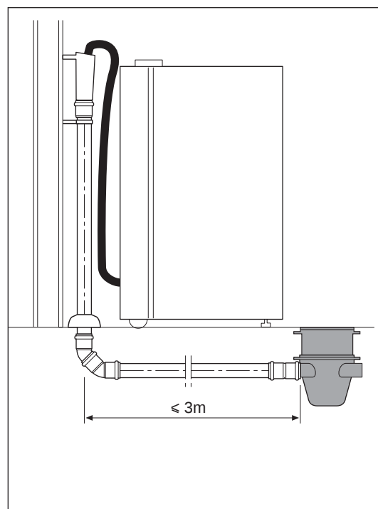
Kuva 85. Pesukoneen liittäminen viemäriverkostoon pesukonesuppilolla.
