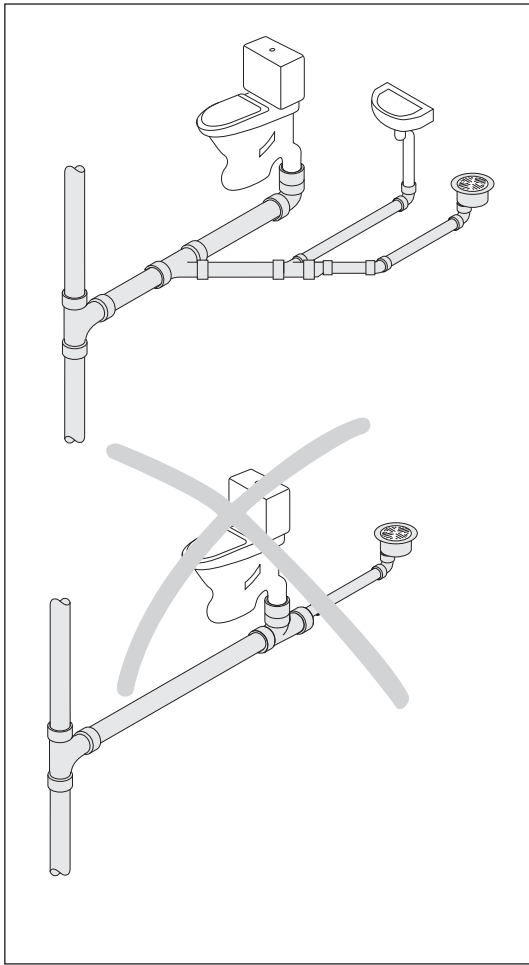
Kuva 86. Kytentäviemärin liittäminen WC-istuimeen tuulettamattomaan viemäriin.
