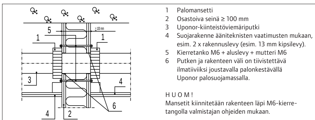
Kuva 110. Esimerkki palomansetin asennuksesta viemärin läpivientiin levyrakenteisen osastoivan seinän pinnalle.
