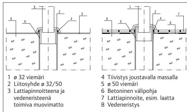
Kuva 89. Esimerkki kytentäviemärin läpiviennistä kostean tilan betonirakenteisessa välipohjassa.
