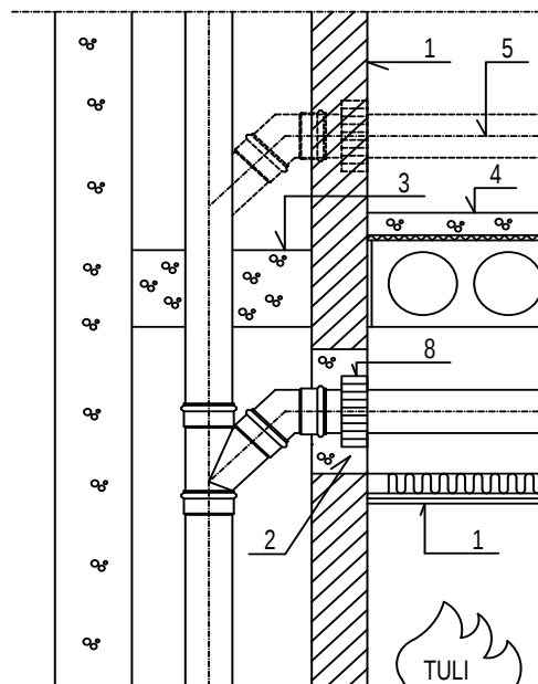
D. Uponor-kiinteistöviemärin palo-osastointi pystykokoojaviemärin suojarakenteella ja suojarakenteen lävistävällä vaakaviemärissä olevalla palomansettilla. Vaakaviemärit välipohjan ylä-/alapuolella.
