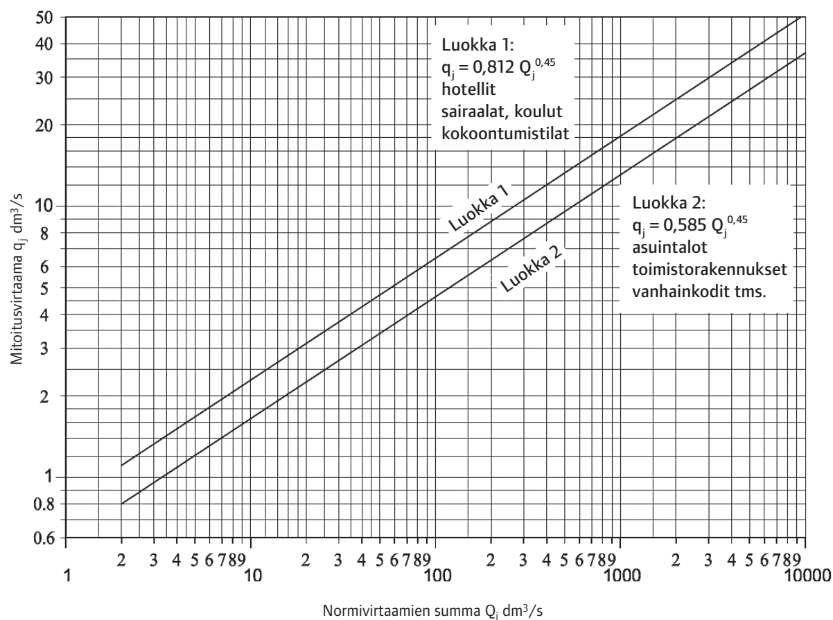
Taulukko 12. Viemärin mitoitusvirtaaman riippuvuus normivirtaamien summasta.
