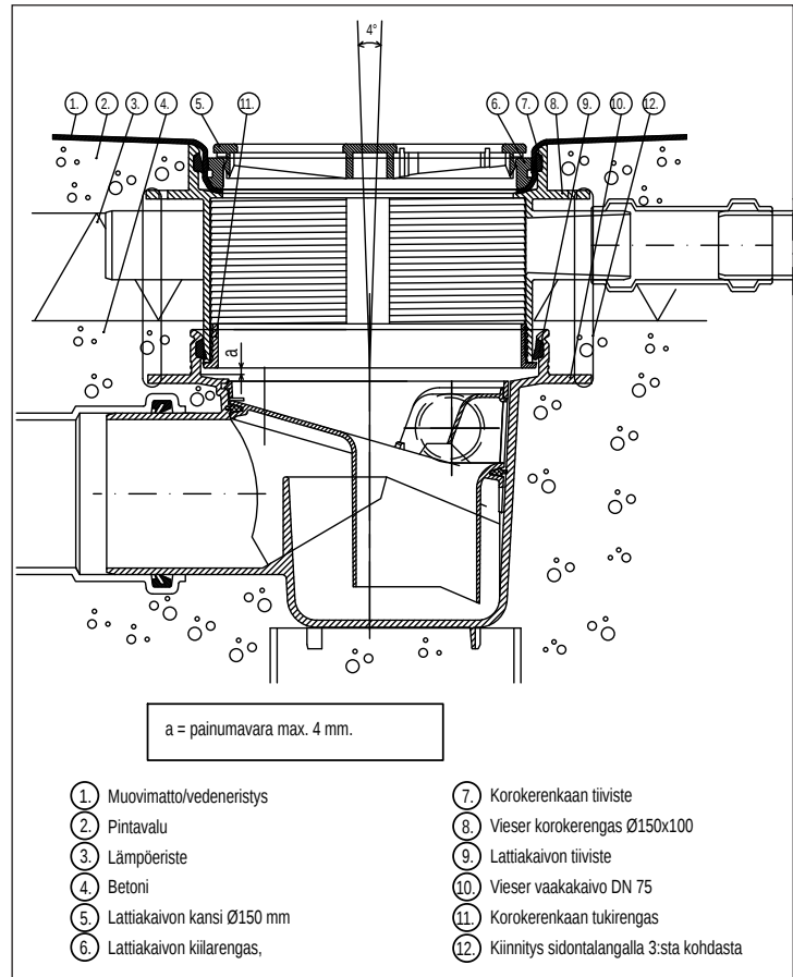
Kuva 97. Vesitiiviin korokerengaan asennus lattiakaivoon betonilattiassa.
