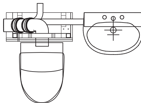
Kuva 56. B2 seinä-WC-elementti V50 keittiö- ja pesuallaskytkenällä.
