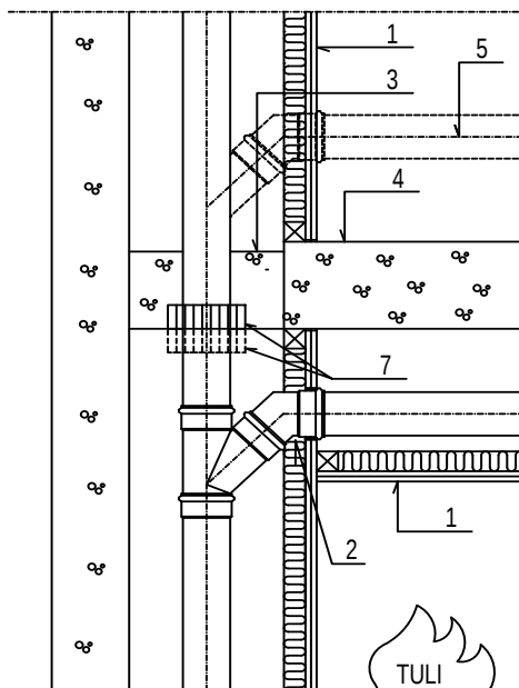
C. Uponor-kiinteistöviemärin palo-osastointi pystykokoojaviemärissä olevalla palomansettilla. Vaakaviemärit betonirakenteisen välipohjan ylä-/alapuolella.
