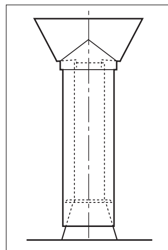
Kuva 40. Tuuletusviemäriin jäätymissuoja tuuletusviemäriin asennettuna.
