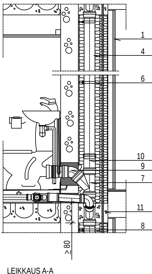
Kuva 8. Esimerkki levyrakenteisesta seinärakenteesta eristetyin Uponor-kiinteistöviemärin yhteydessä äänitasovaatimuksella 33 dB(A). EI 30.
