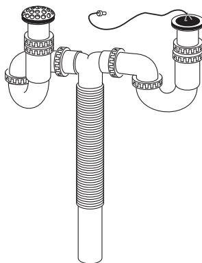
Kuva 117. Saneeraus-vesilukko.
