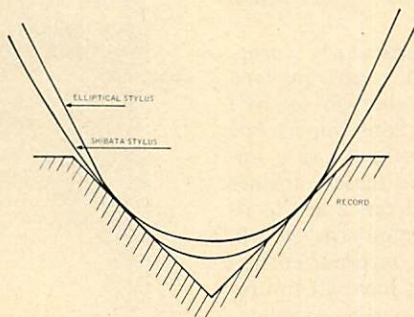
Fig. 6—Shibata stylus.
