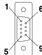
CN-2 (D-Sub 9-pin side)
