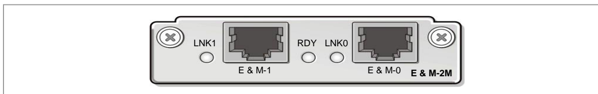
Figure 28. E & M-2M Mini Module
