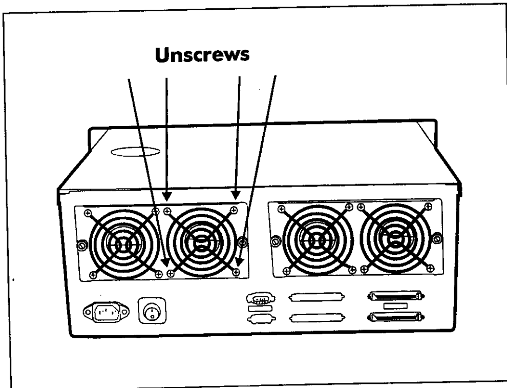
Figure : Swap Cooling Fan ( swap with a new Fan )
