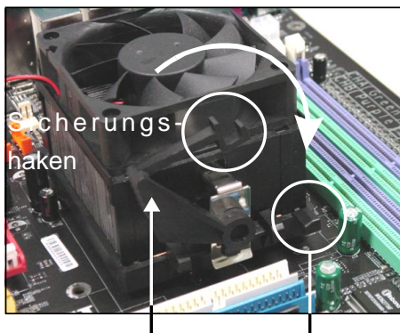
Sicherungshaken Sicherungshebel Sicherungsbolzen
