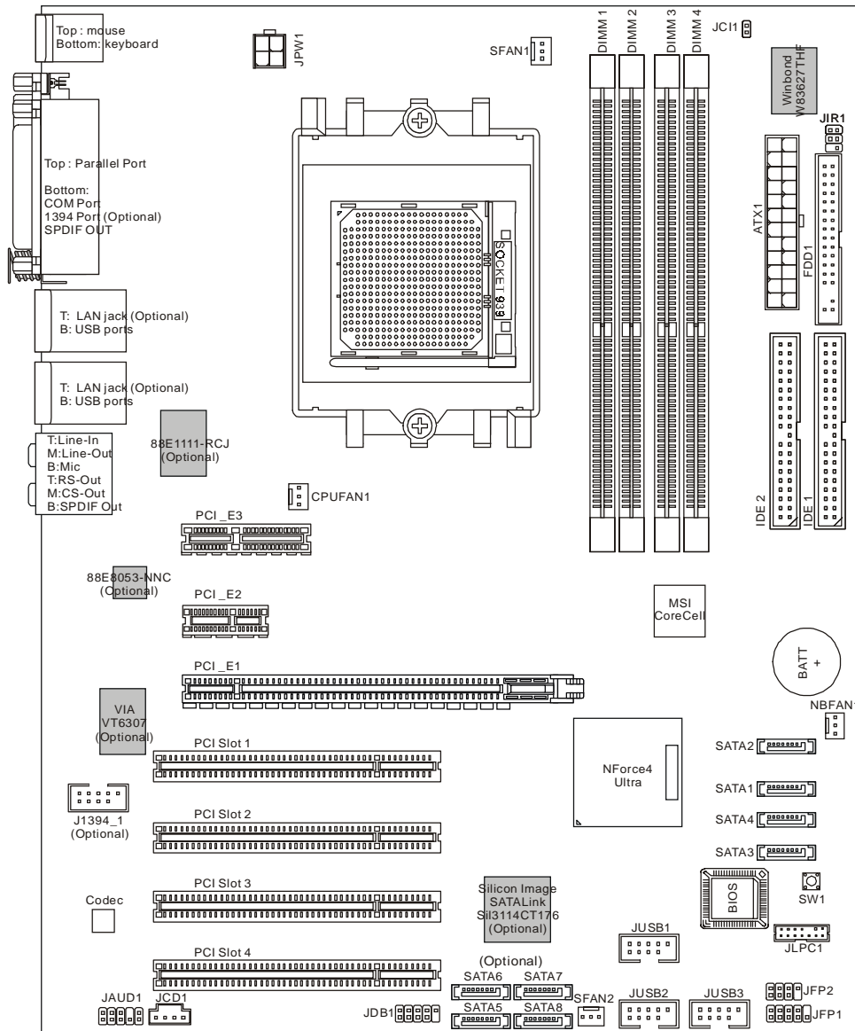
K8N Neo4 Platinum (MS-7125 v1.X) ATX Mainboard
