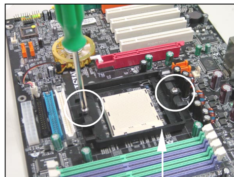
Rückhaltemechanismus
