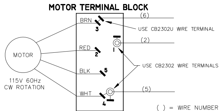
(SK 737W2 Motor Wiring)
