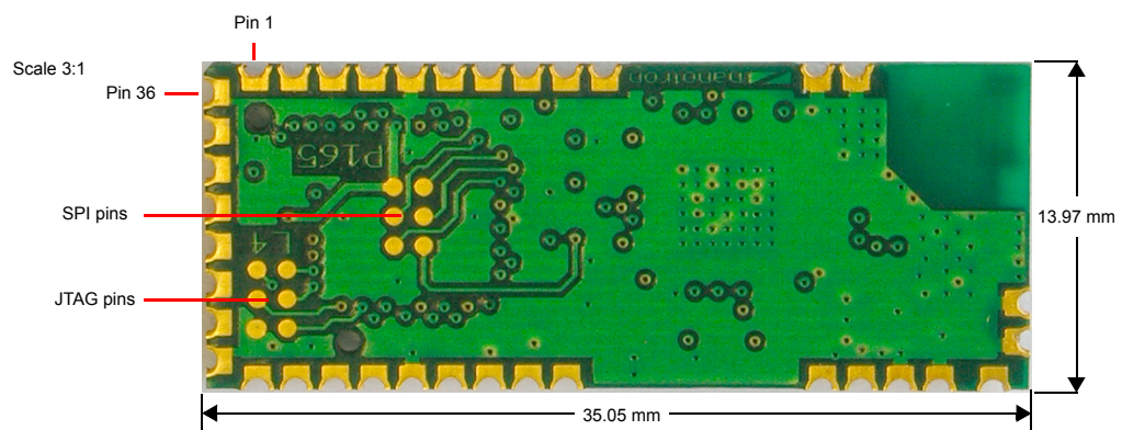
Figure 3: nanoLOC AVR Module - pad side
