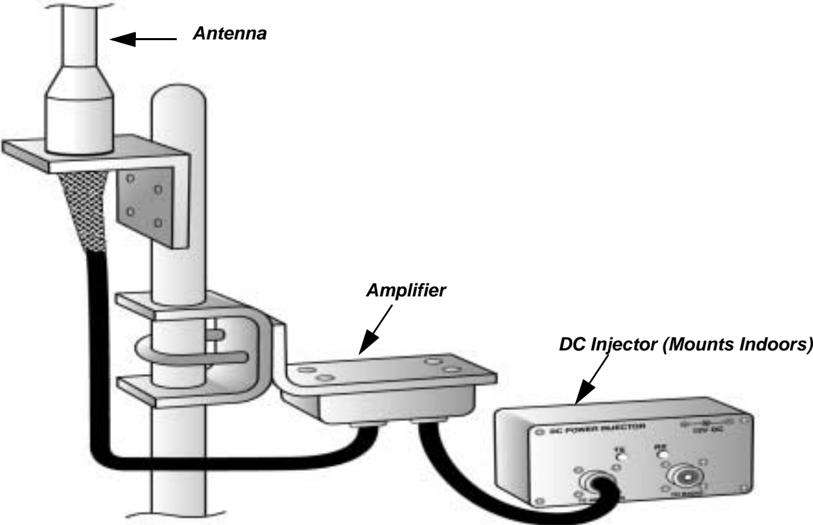
Amplifier Wiring
