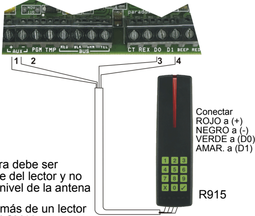
Figura 2: Conexión del R915
