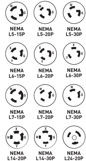
20 & 30A Plug
