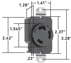
30A Receptacle
