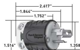
15A Plug
