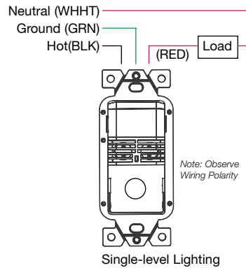
Sensor Wiring
