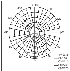
Standard 6000K, 150W Light LPL04-C60-150W
