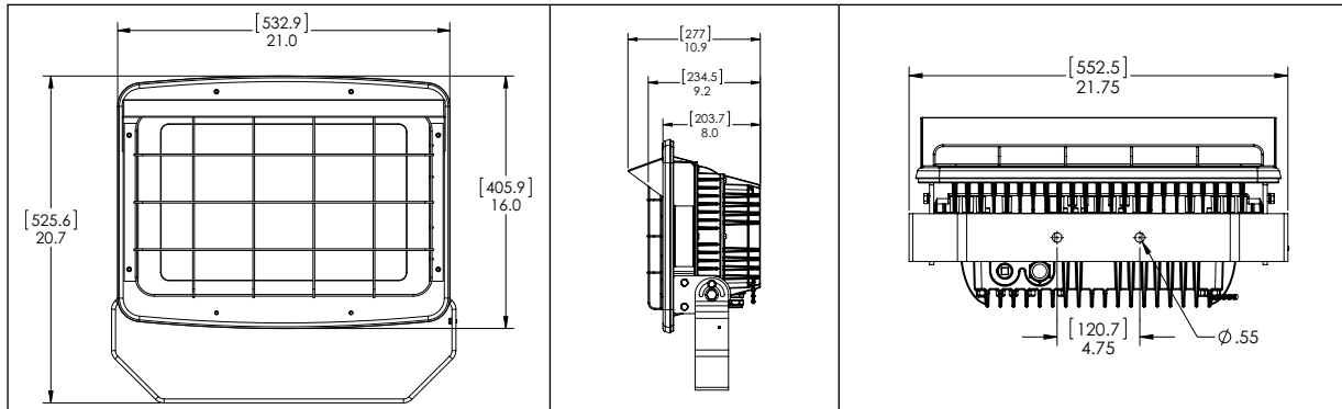
PFM25L Model
