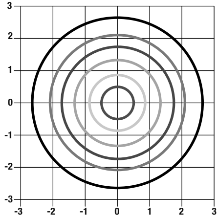
ISOFOOTCANDLE CHART Footcandle Values for Isofootcandle Lines
