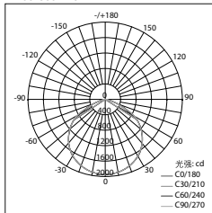
Standard 6000K, 125W Light LPL06-C60-125W
