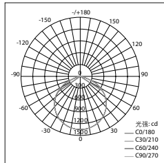
Standard 6000K, 85W Light LPL04-C60-85W
