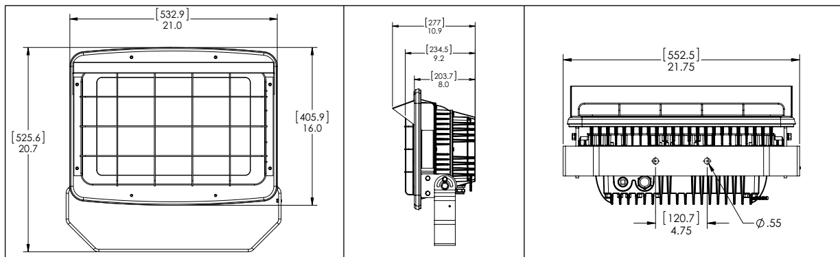
PFM25L Model
