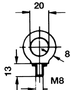
Eyebolt A2
