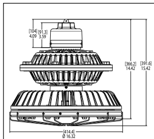
Pendant Mount
