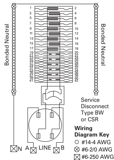
Catalog Number—MBE3042B225BF
