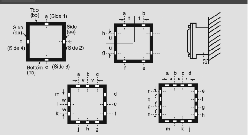
CONDUIT ARRANGEMENT DIAGRAMS
