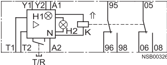
3RN10 13-... 0
