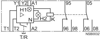
3RN10 13-... 1 (bistable)
