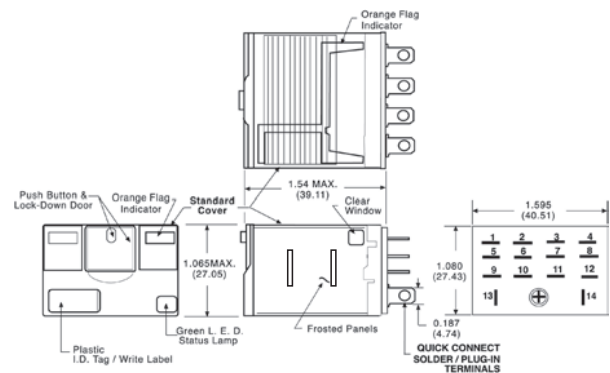
3TX7117 4PDT
