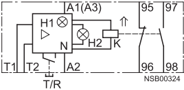
3RN10 13-... 0
