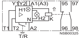
3RN10 12 1)
