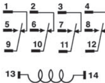
3TX7112-1L, -1D
