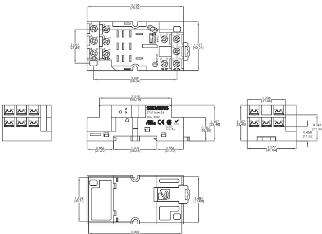
3TX7144-4E8
