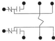
3TX7130 DPDT
