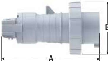
32A PLUG
