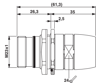
UC-0000000Q0DU (Axial O-ring)
