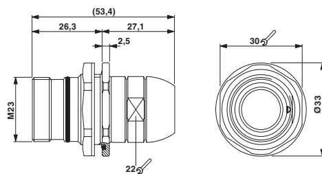
RC-0000000Q0FZ Axial O-ring
