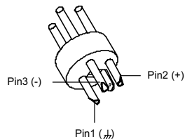
XLR, symmetrisch
