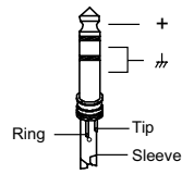
Stereoklinke, unsymmetrisch
