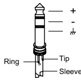
Stereoklinke, symmetrisch
