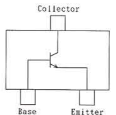
2SC2712GR (LG) (Q3006, 3010, 3011 3015, 3016, 3017 3020)
