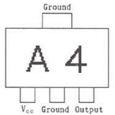
M51943BML (A4) (Q3023)
