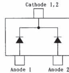
1SS184 (B3) (D7201)
