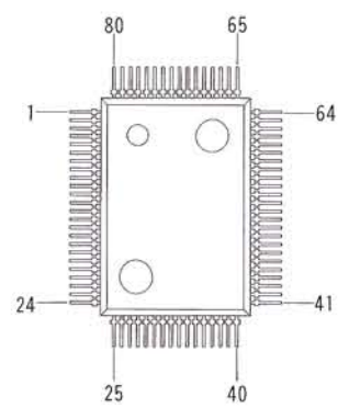
M37450E4FP MY-021 (Q6517)
