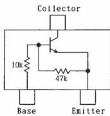
FA1A4P (L34) (Q7202)
