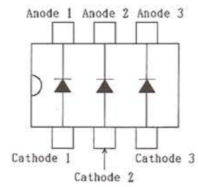
IMN10 (N10) (D3014, 3026, 3029 3033, 3044)
