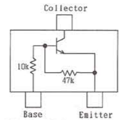
FA1A4P (L34) (Q3001, 3002, 3007 3012, 3019, 3021 3028, 3030, 3035 3036, 3039)
