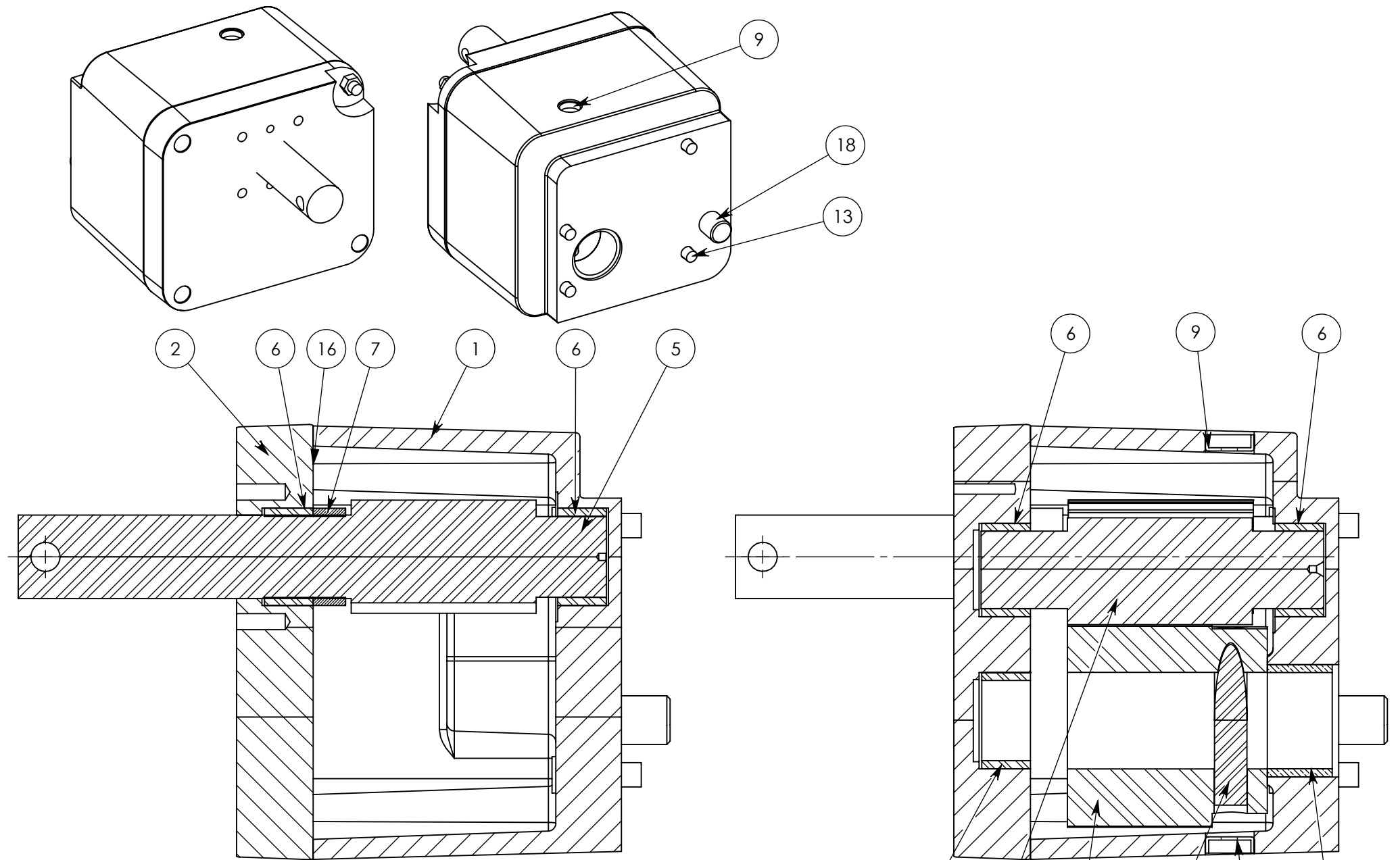
SECTION D-D
