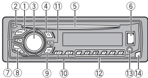
DEH-X4600BT
