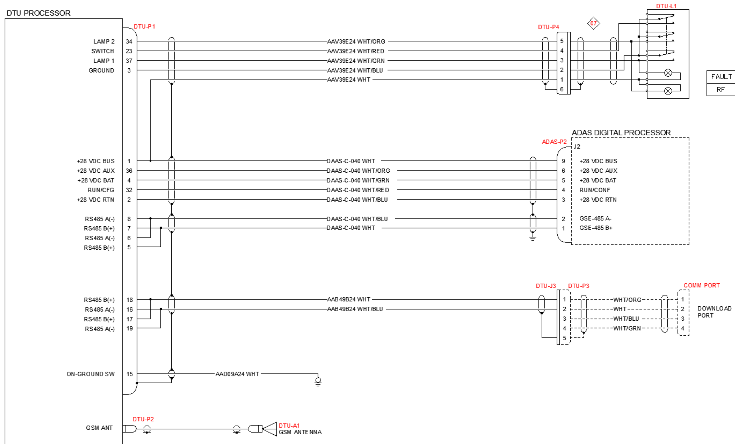
Figure B- 19: DTU / ADAS d Wiring Schematic
