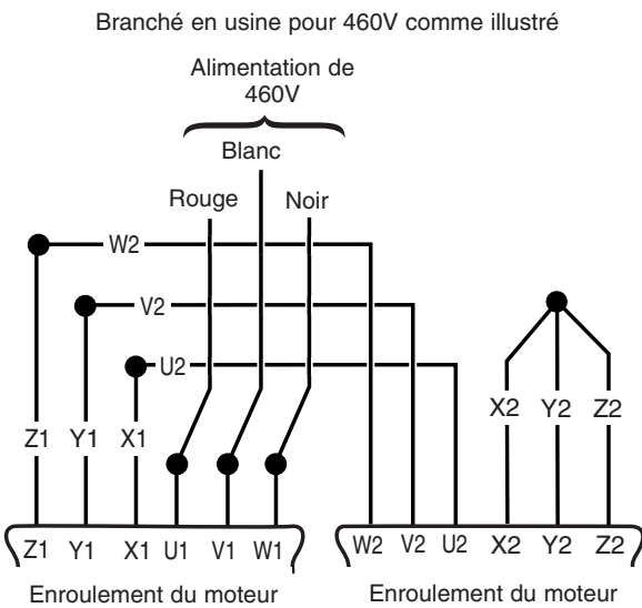
Figure 3 : Connexions de câblage triphasé de 460 Volts
