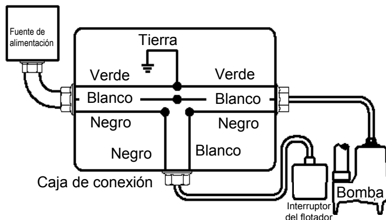
Fig. 5 – Cableado directo de bombas automáticas monofásicas de 115 V o 208-230 V
