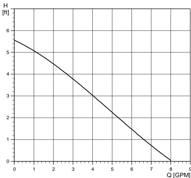
UP 15-10 F
