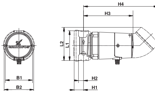
UP 10-16 B5/BN5
