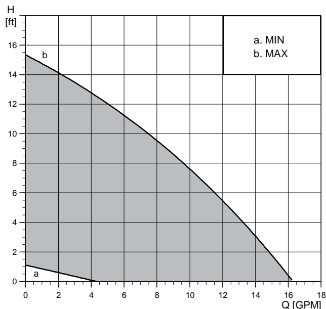
UP 15-42 F/VS
