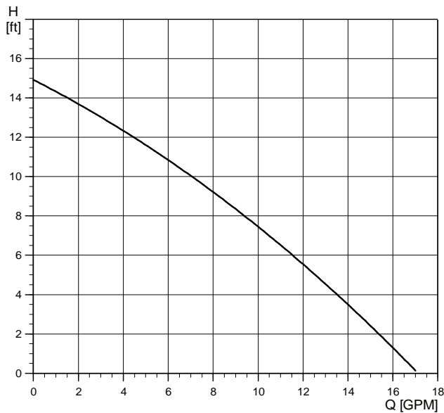
UP 15-42 F
