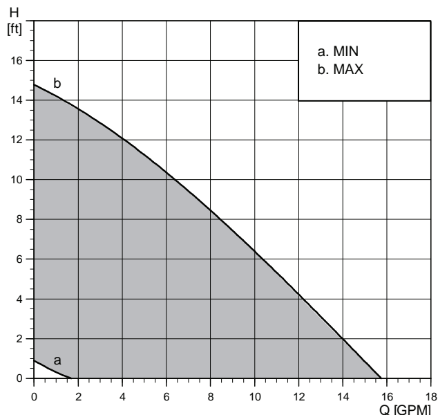
UP 15-42 FC/MR
