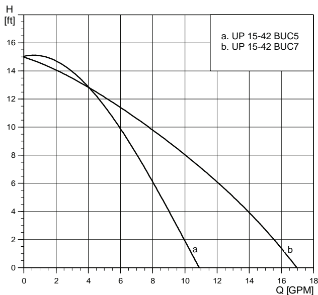
UP 15-42 BUC5
