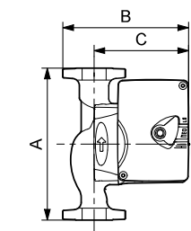
UPS 15-58 FC
