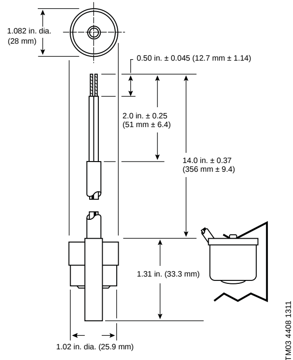
Fig. 14 AquaStat dimensions
