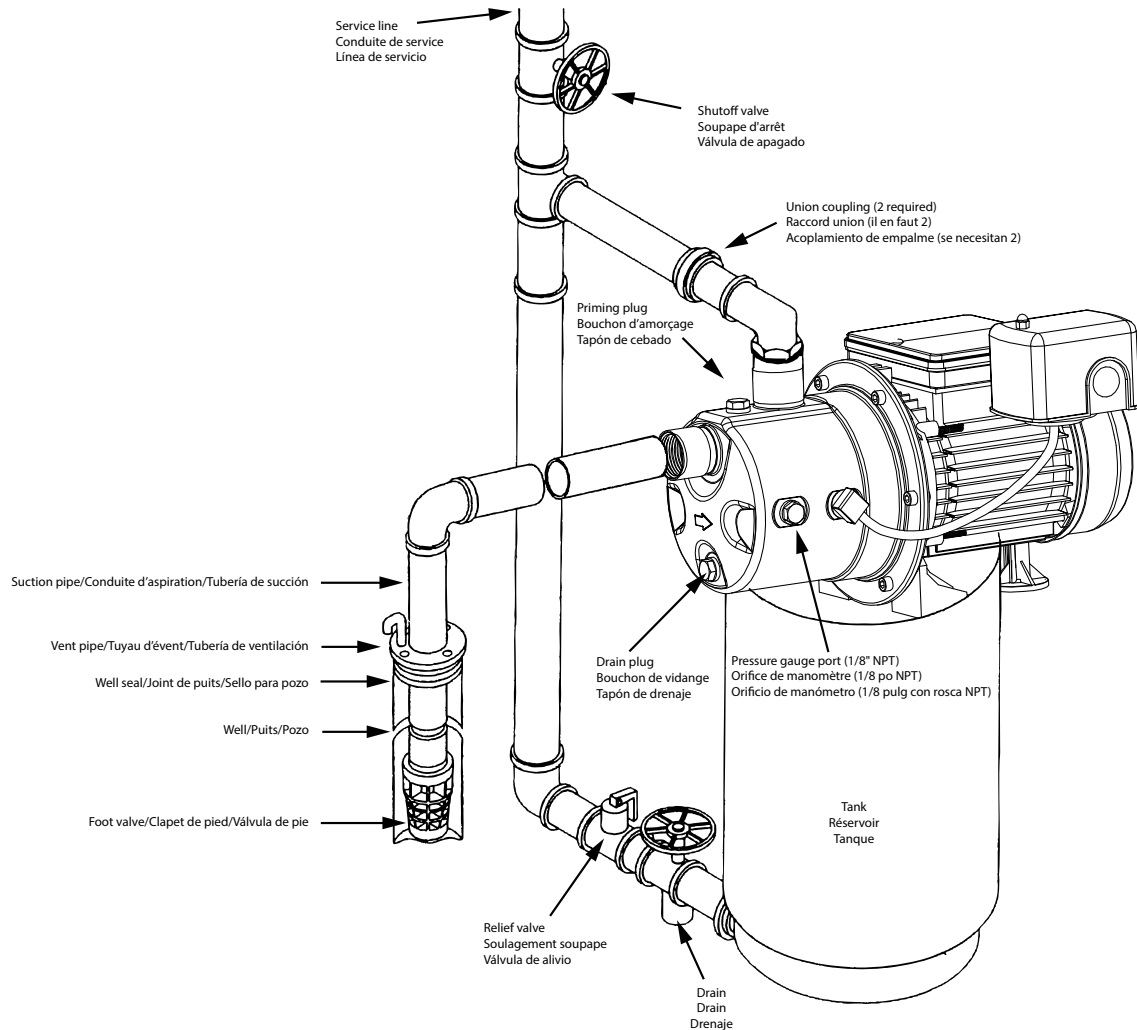
FIGURE 7 • FIGURE 7 • FIGURA 7 SHALLOW WELL - TANK-MOUNTED SYSTEM (WITH FOOT VALVE) • Puits peu profond, système de réservoir monté (avec clapet de pied) • POZO POCO PROFUNDO, SISTEMA MONTADO EN TANQUE (CON VÁLVULA DE ASPIRACIÓN)
