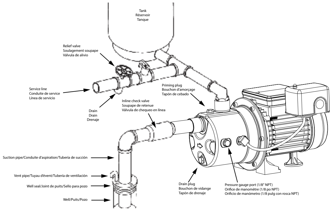
FIGURE 6 • FIGURE 6 • FIGURA 6 SHALLOW WELL (WITH INLINE CHECK VALVE) • Puits peu profond (avec clapet anti-retour en ligne) • POZO POCO PROFUNDO (CON VÁLVULA DE RETENCIÓN EN LÍNEA)
