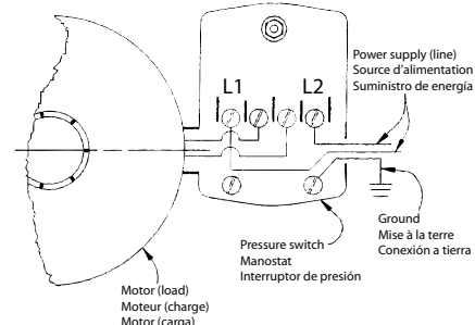
FIGURE 2 • FIGURE 2 • FIGURA 2 ELECTRICAL CONNECTIONS • CONNEXIONS ÉLECTRIQUES • CONEXIONES ELÉCTRICAS
