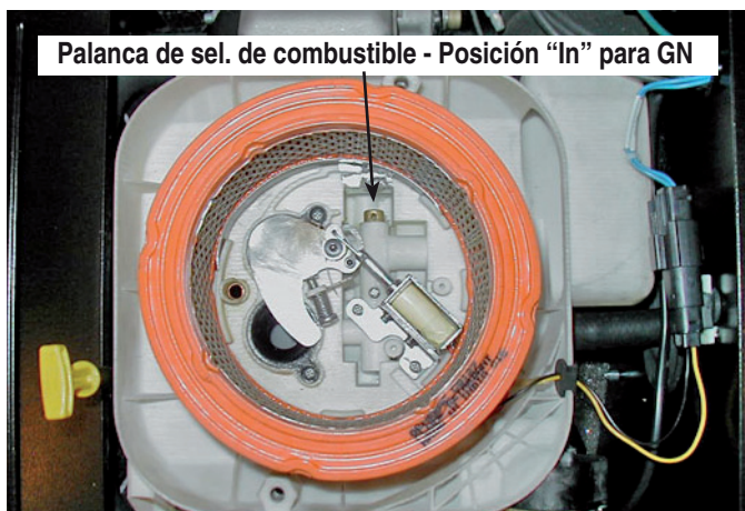
Figura 1.8 - 14, 17, y 20kW, GT-990/GT-999 (cubierta de caja de aire retirada)
