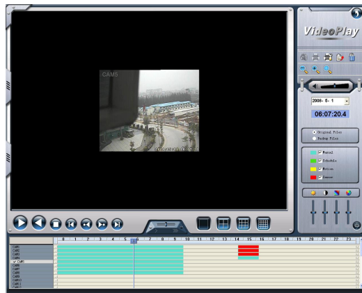
Figure7-18Example: zoomed out
