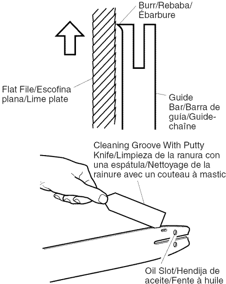
Figure 18 - Guide Bar Maintenance Figura 18 - Mantenimiento de la barra de guía Figure 18 - Entretien de la guide-chaîne
