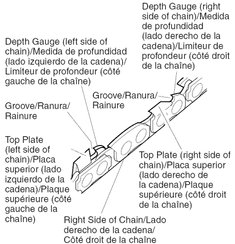
Figure 20 - Chain Part Locations Figura 20 - Posición de las partes de la cadena Figure 20 - Emplacement des pièces de la chaîne
