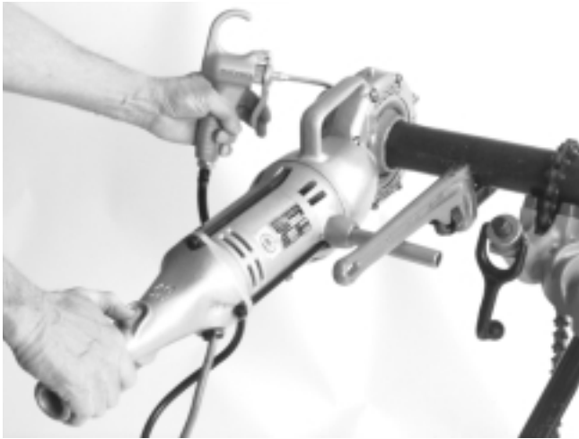
Figura 6 – Roscado empleando una llave de tubo como brazo de soporte
