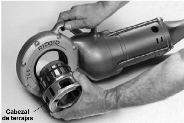
Figura 3 – Instalación del Cabezal de terrajas No. 12-R
