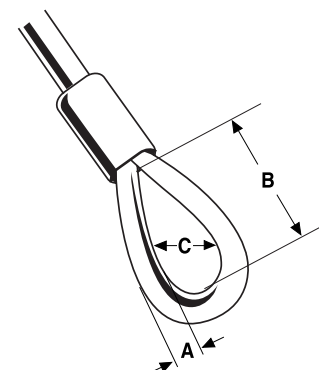
Loop Dimensions
