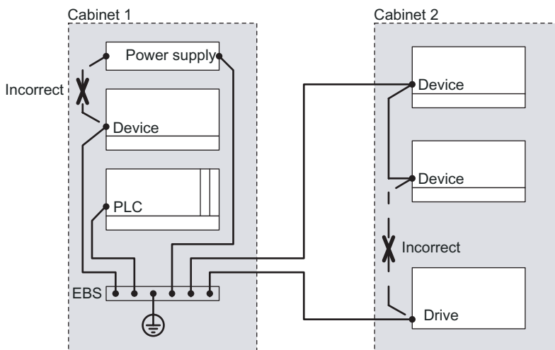
Figure 4-27 Equipotential bonding (EBS = Equipotential bonding strip)
